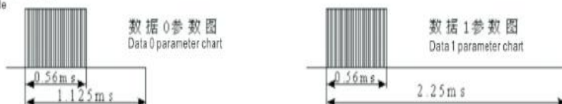
发码数据参数示意图 Sketch map of hair code
