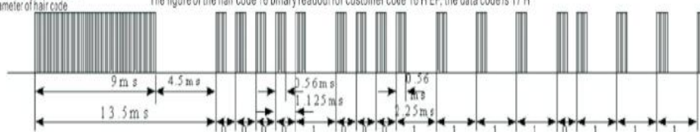
发码时间参数图 Time parameter of hair code
