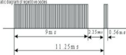
发码数据参数示意图 Sketch map of hair code
