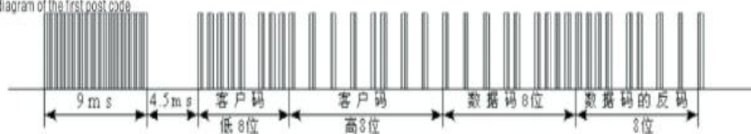
发码时间参数图 Time parameter of hair code
