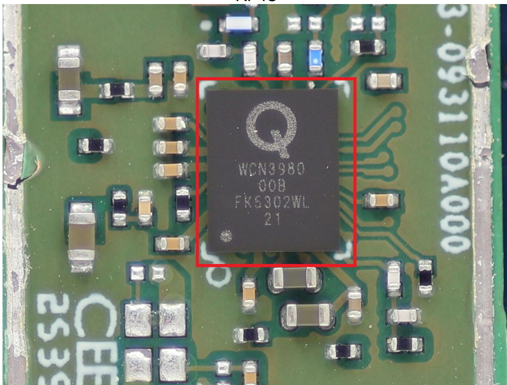
RF IC
