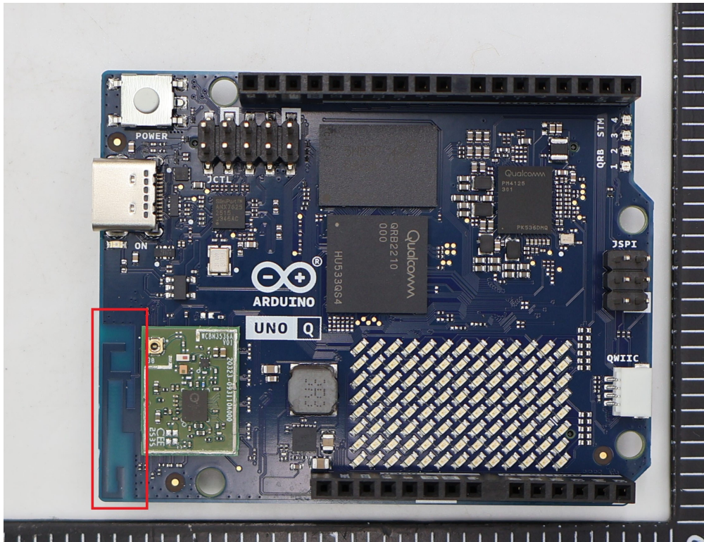
Antenna
