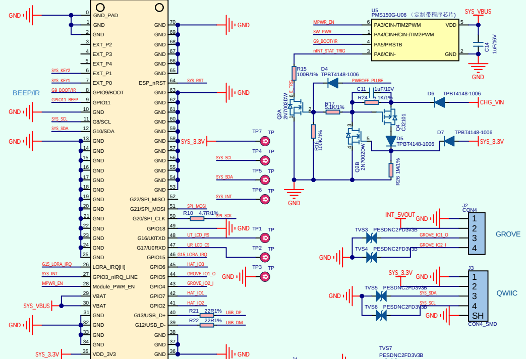
U8 M5Stack_Lora_C6模组
