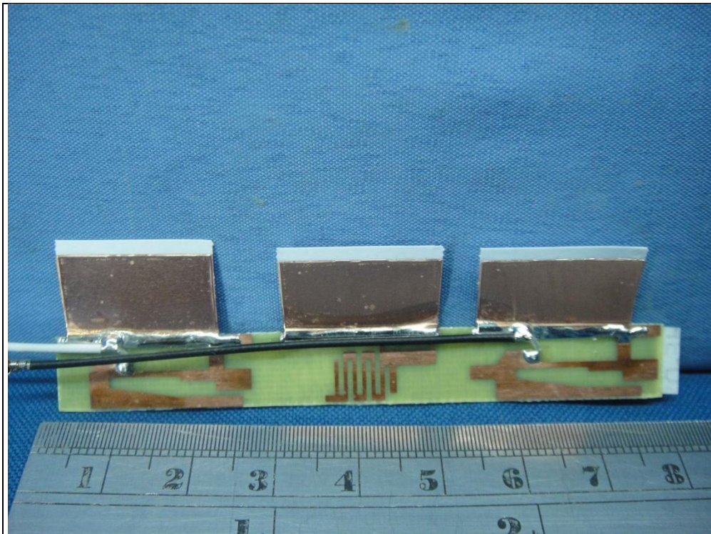
Antenna set 2
