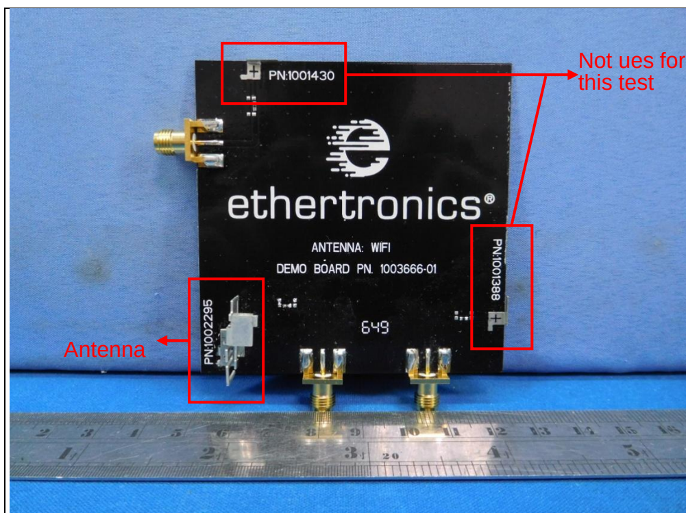
Antenna set 4
