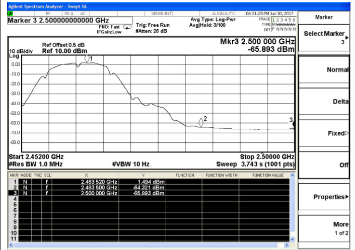
802.11b High channel(Average)
