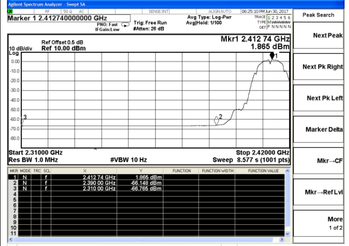
802.11b Low channel(Average)
