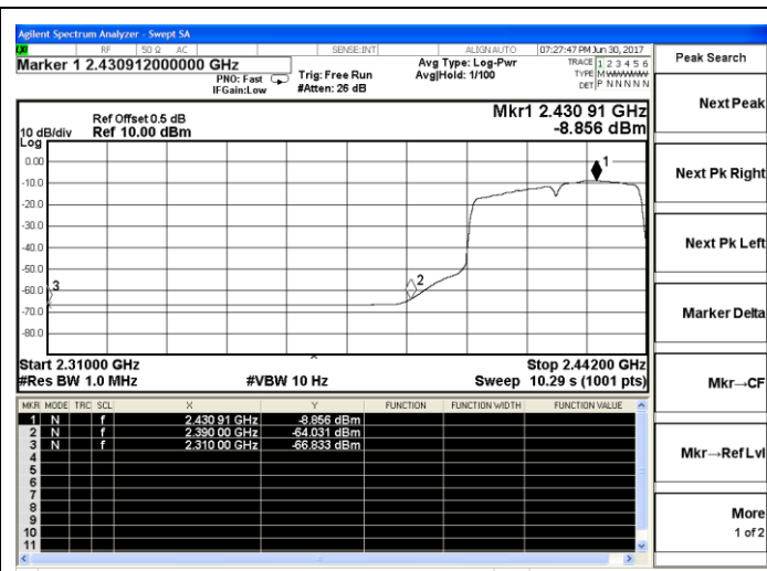
802.11n-HT40 Low channel(Average)
