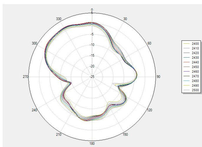
2400-2500MHz-Phi 90
