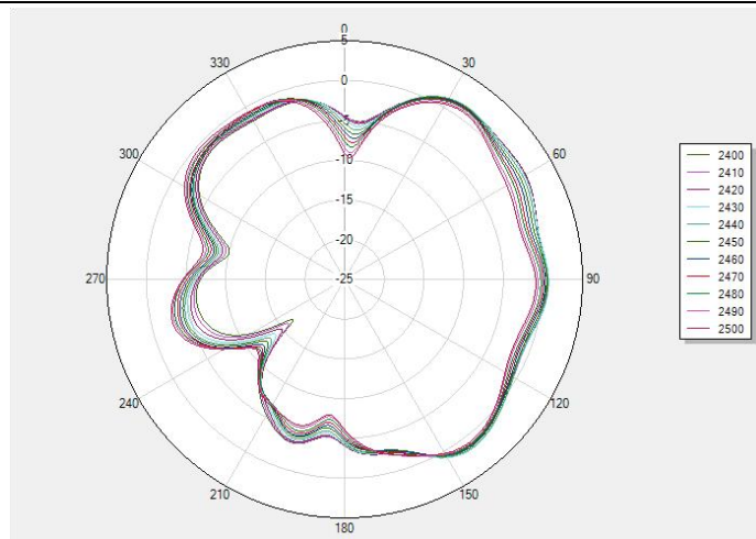
2400-2500MHz-Phi 0
