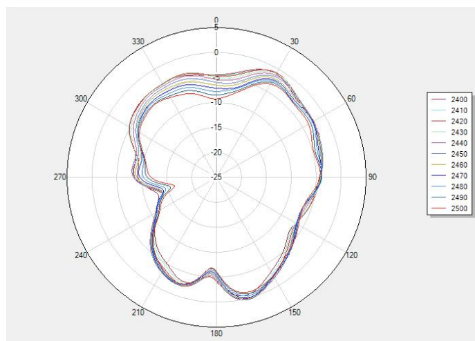
2400-2500MHz-Phi 90
