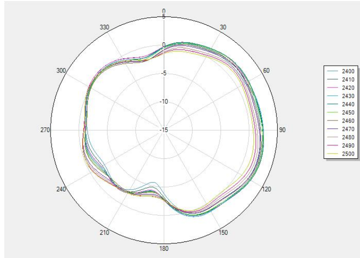
2400-2500MHz-Theta 90
