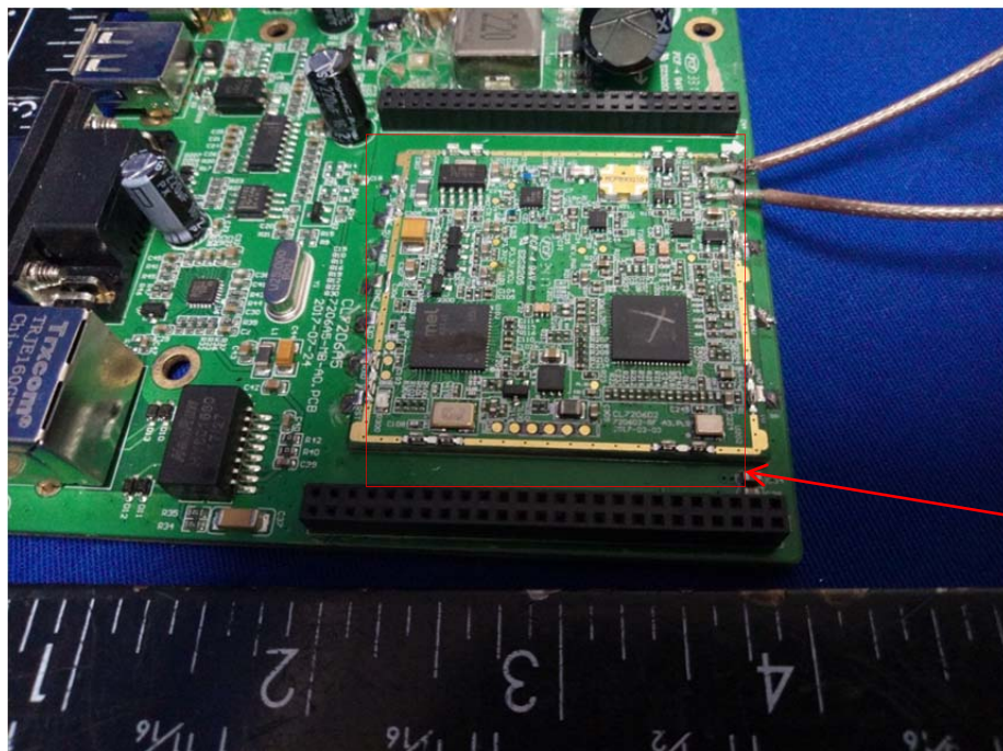
RFID Module
