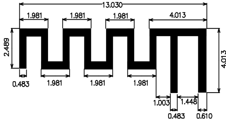
CS61008-ANTENNA
