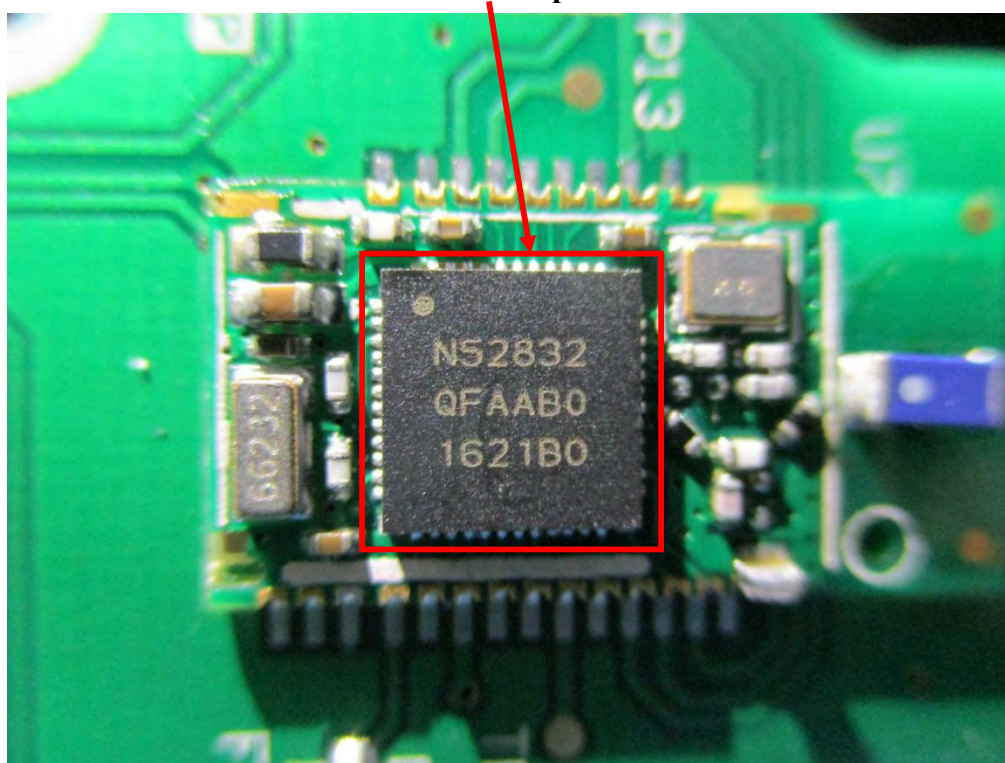
BLE IC – Top View
