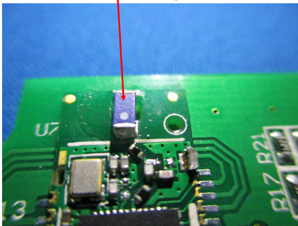
BLE Antenna – Top View
