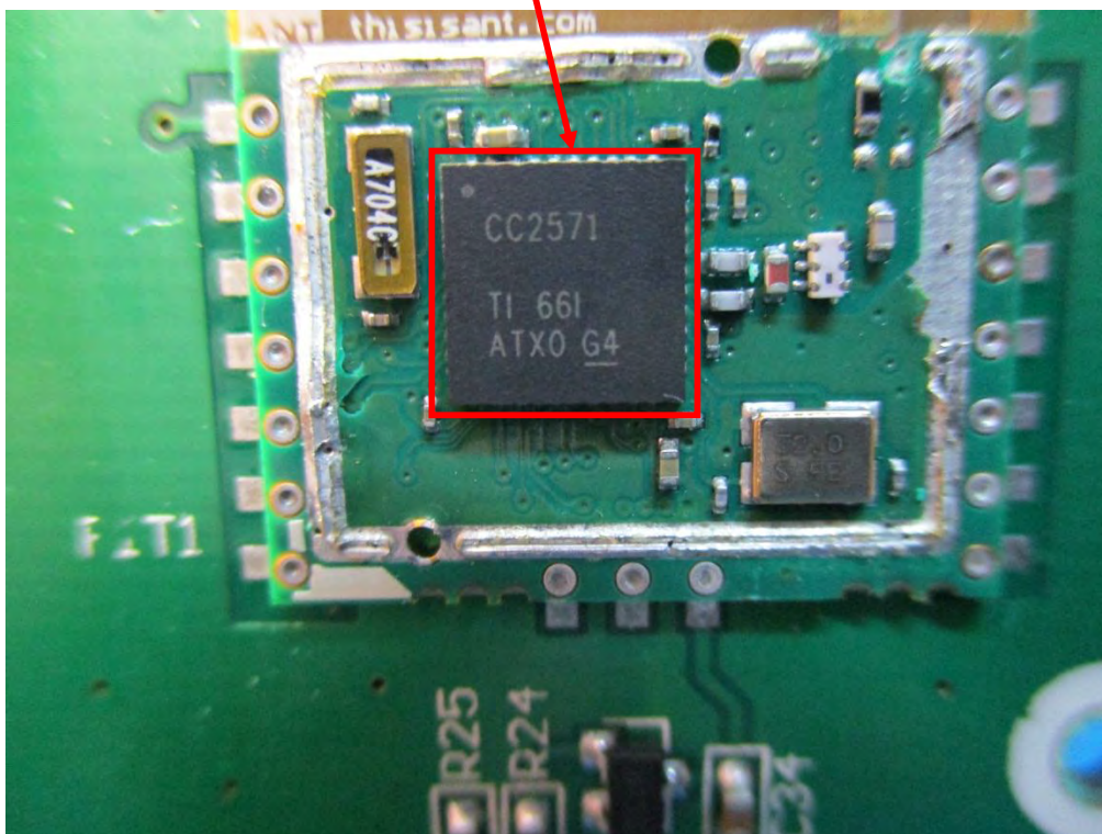
ANT+ IC - Top View
