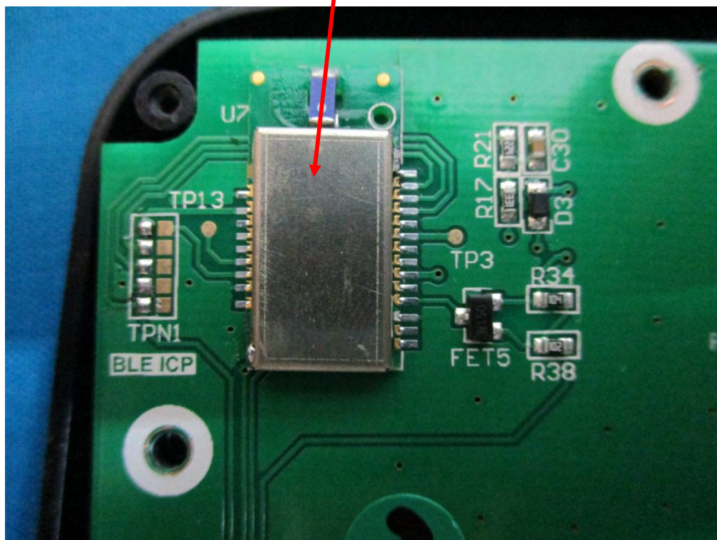
BLE Module – Top View
