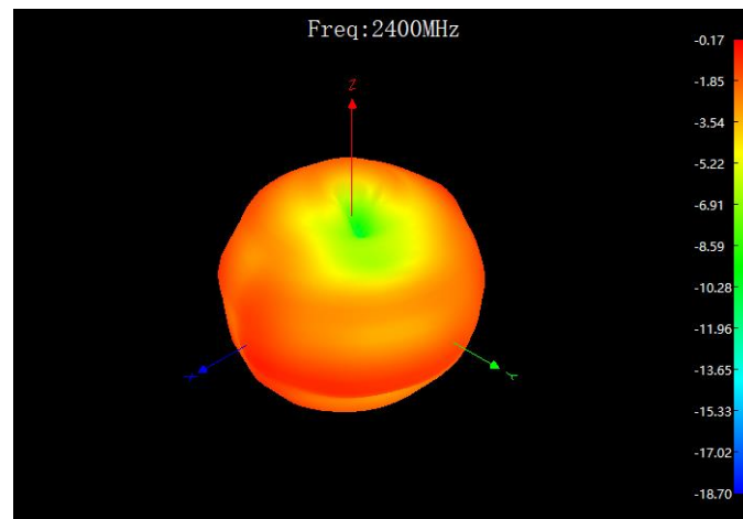
2450MHz 3D
