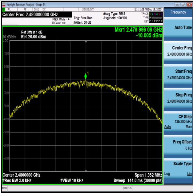
BLE_500K-Ant1-2480-PASS
