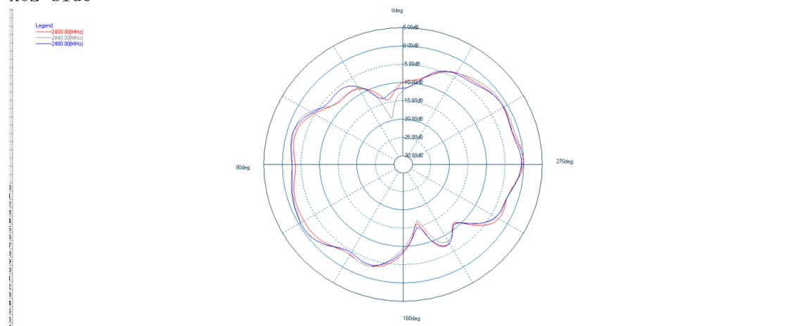
XOZ side
