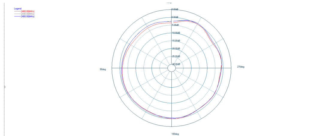
XOY side
