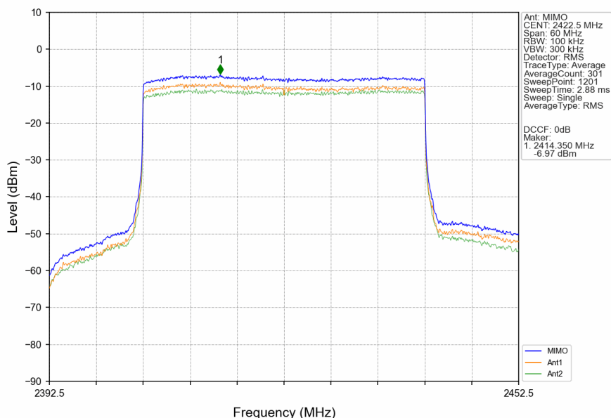
40M_LCH_2422.5MHz_MIMO_NTNV
