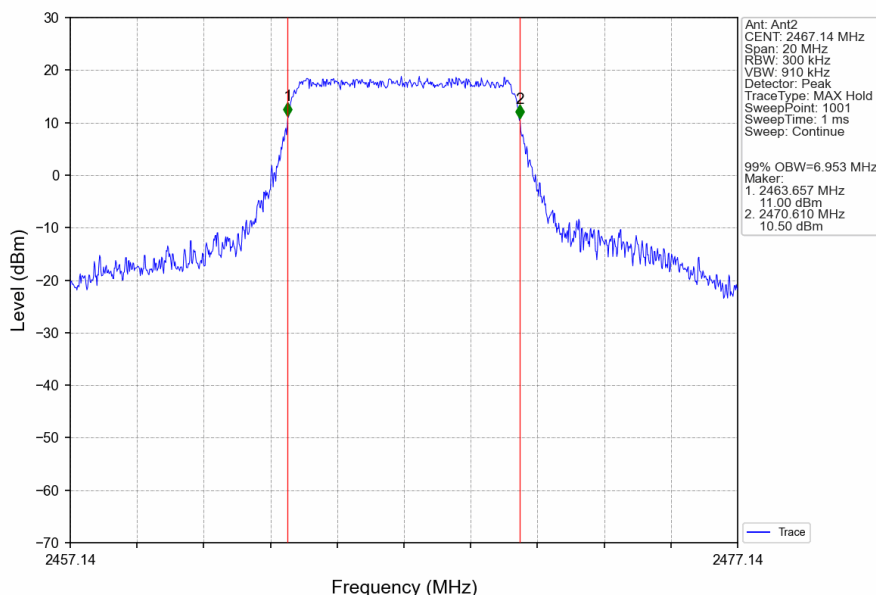
10M_HCH_2467.14MHz_Ant2_NTNV
