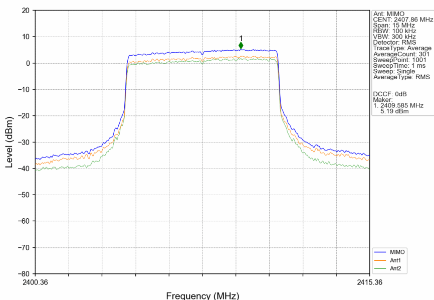
10M_LCH_2407.86MHz_MIMO_NTNV
