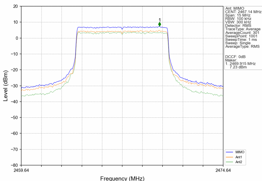
10M_HCH_2467.14MHz_MIMO_NTNV
