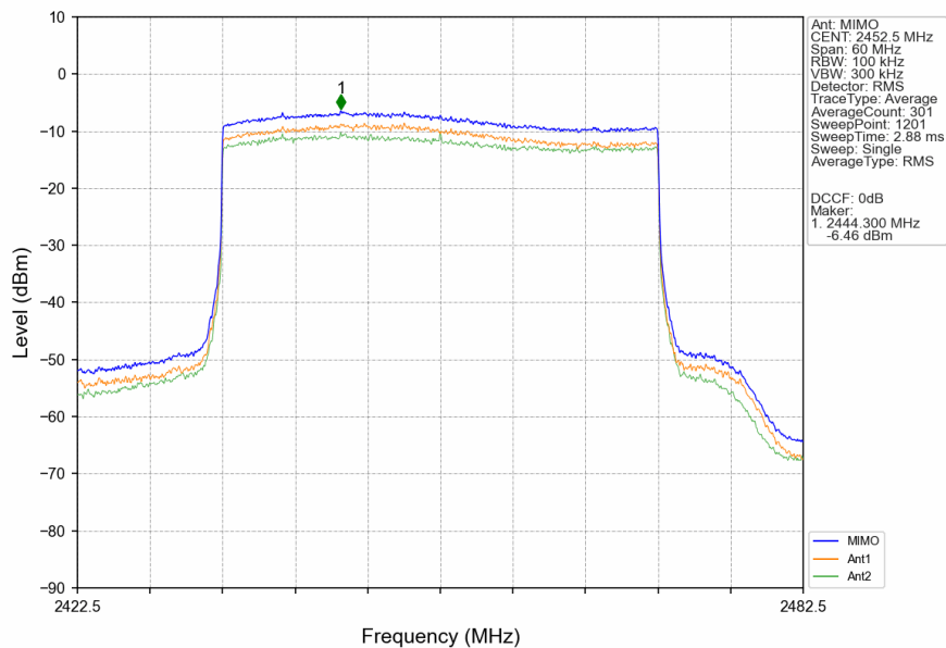
40M_HCH_2452.5MHz_MIMO_NTNV
