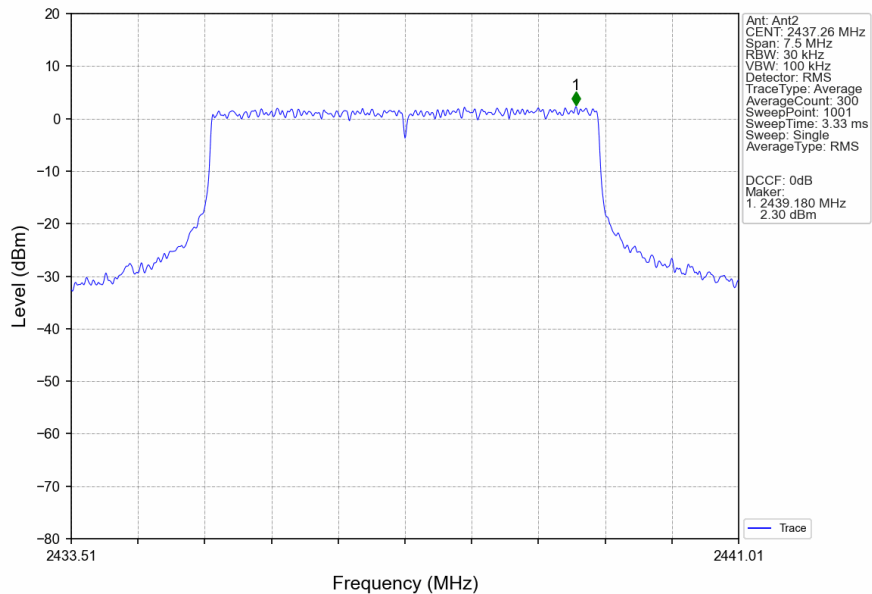
5M_MCH_2437.26MHz_Ant2_NTNV
