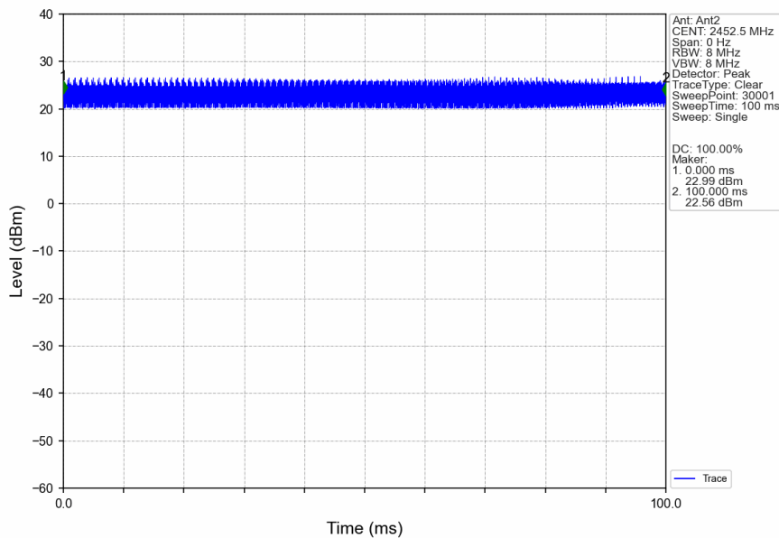
40M_HCH_2452.5MHz_Ant2_NTNV
