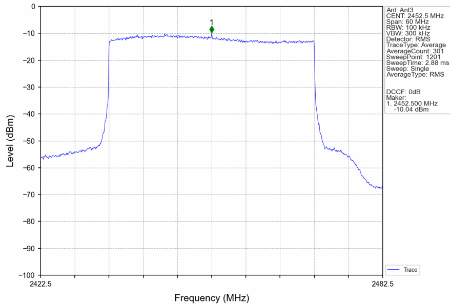
40M_HCH_2452.5MHz_MIMO_NTNV
