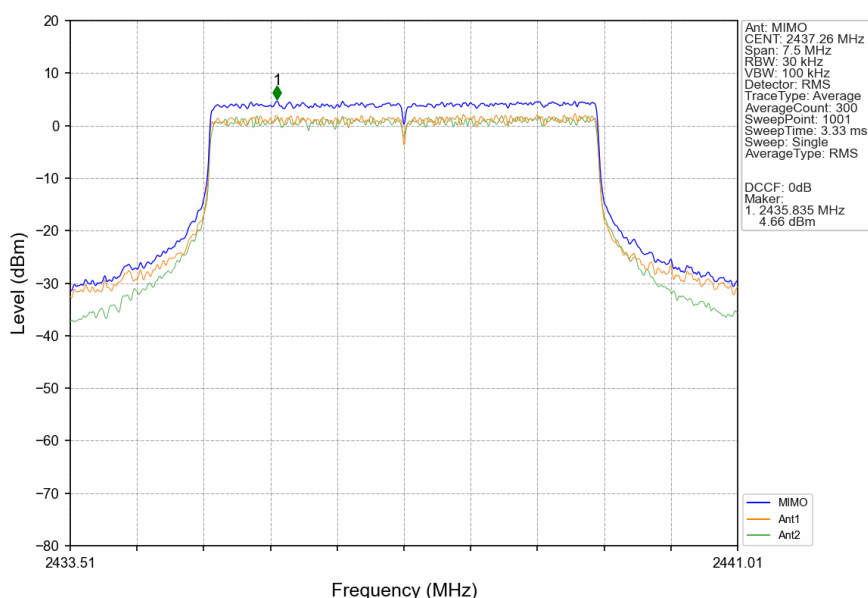
5M_MCH_2437.26MHz_MIMO_NTNV
