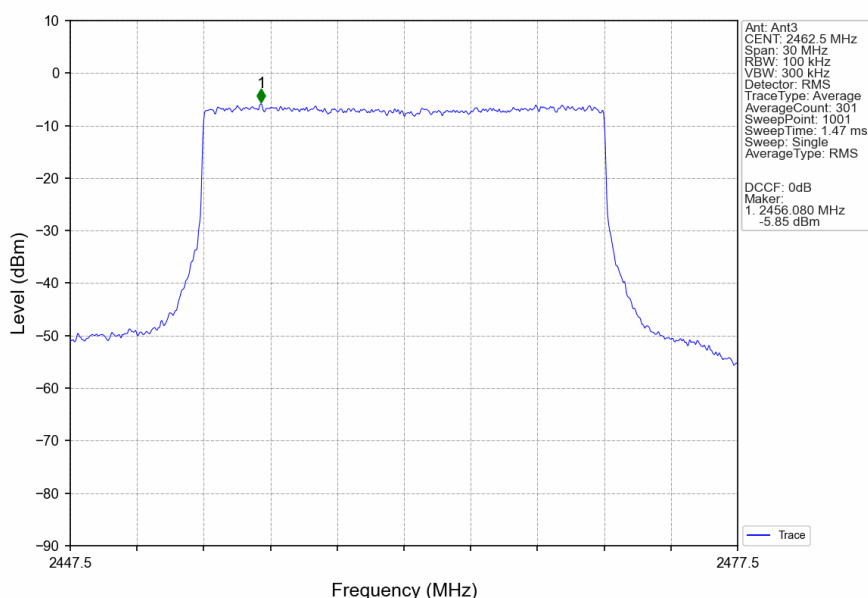
20M_HCH_2462.5MHz_Ant3_NTNV
