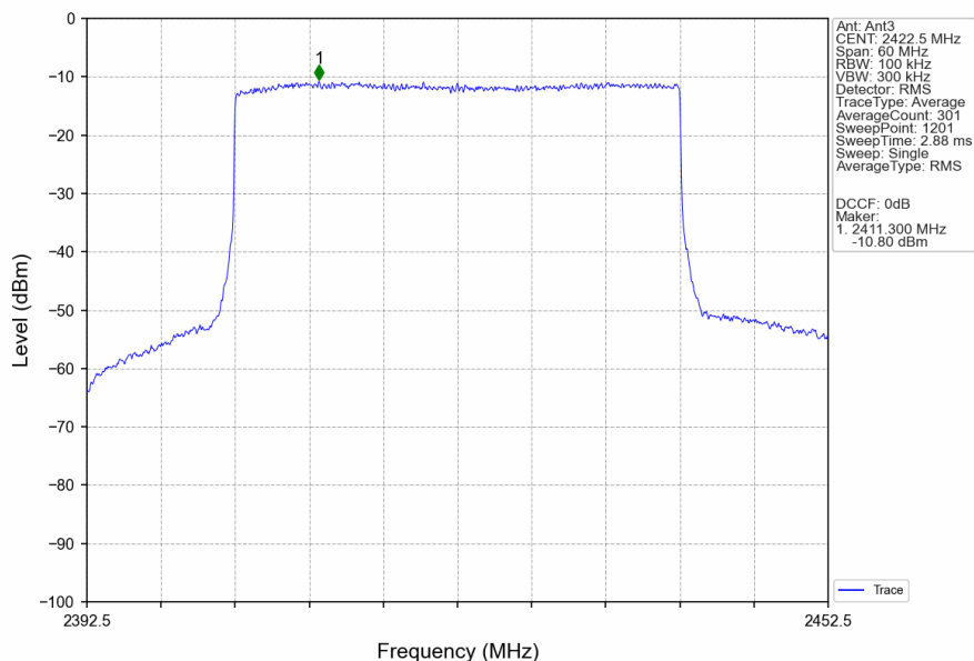
40M_LCH_2422.5MHz_MIMO_NTNV
