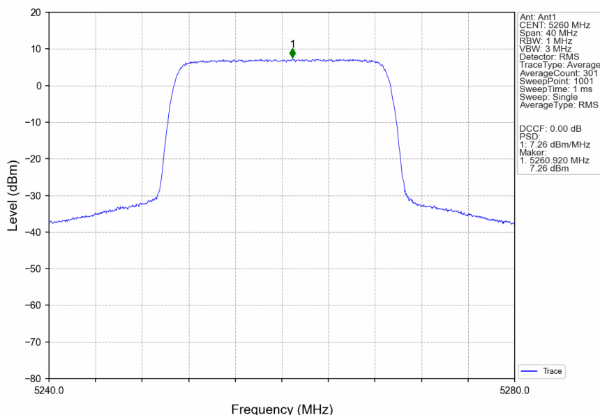
5G 20M B2A_LCH_5260MHz_Ant1_NTNV
