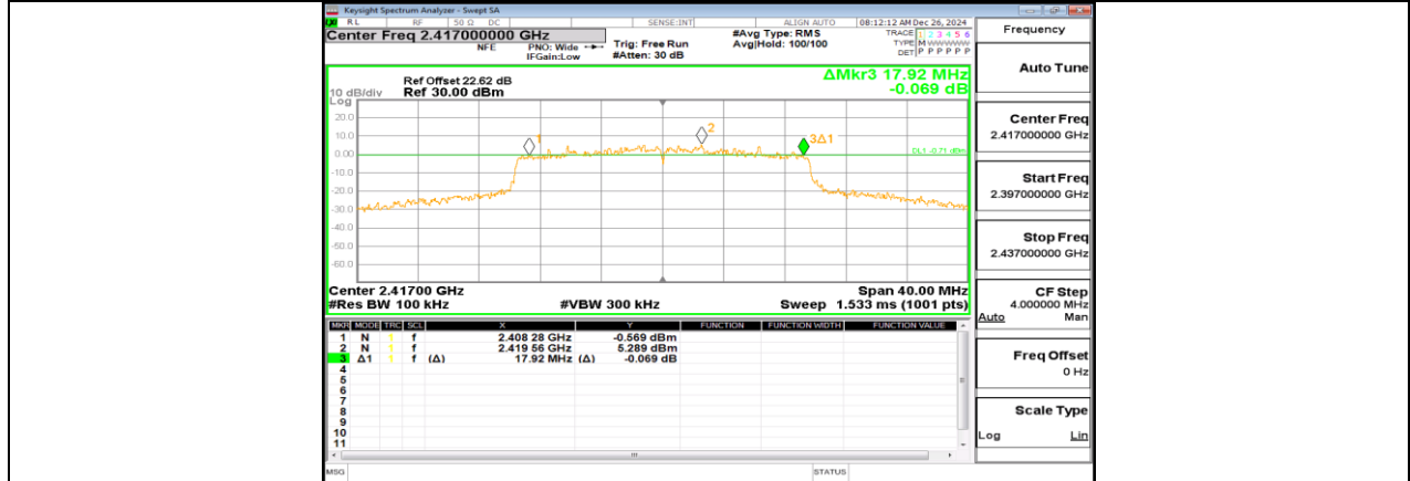
11AX20MIMO_Ant1_2417
