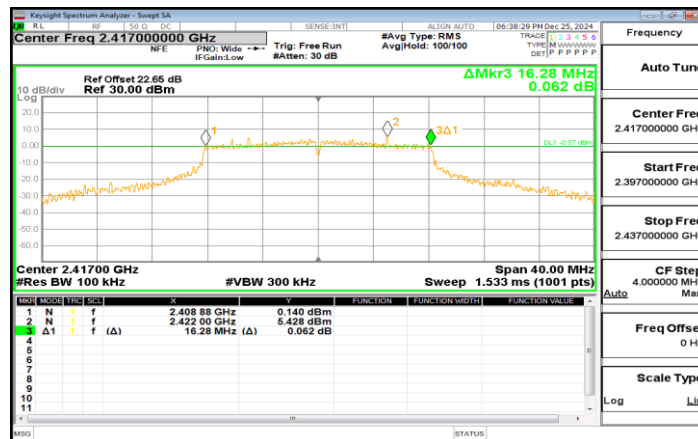
11G-CDD Ant2 2417
