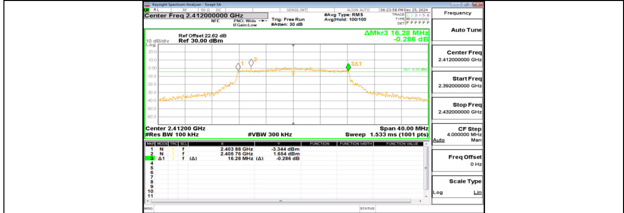
11G-CDD Ant1 2412
