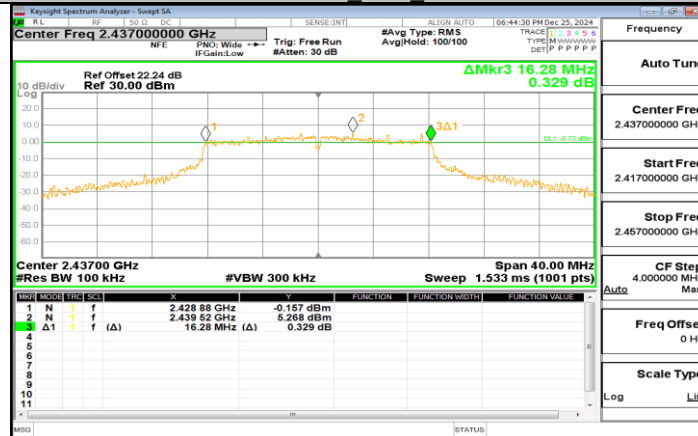
11G-CDD Ant1 2437
