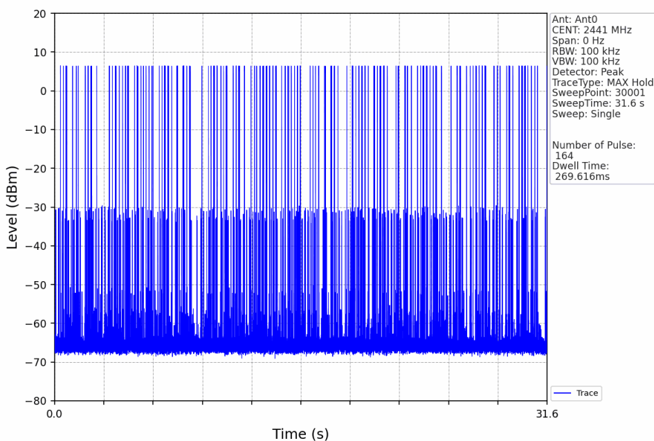
Pi/4DQPSK_2DH3_HOPP_Ant0_NTNV
