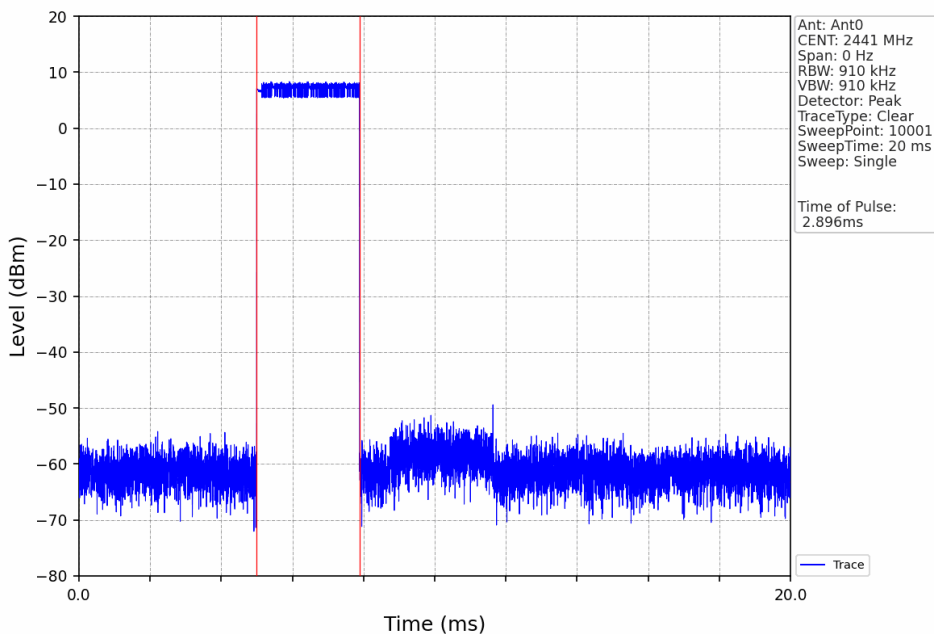
Pi/4DQPSK_2DH5_HOPP_Ant0_NTNV
