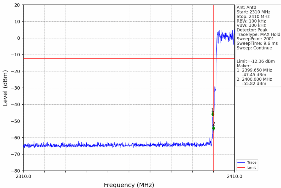
Pi/4DQPSK_2DH5_HOPP_Ant0_NTNV
