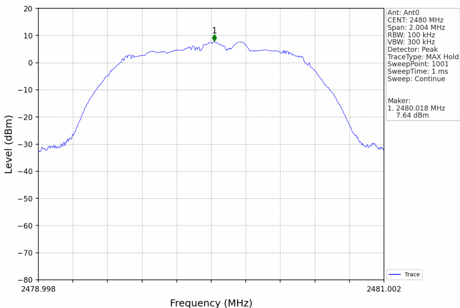
Pi/4DQPSK_2DH5_HCH_2480MHz_Ant0_NTNV
