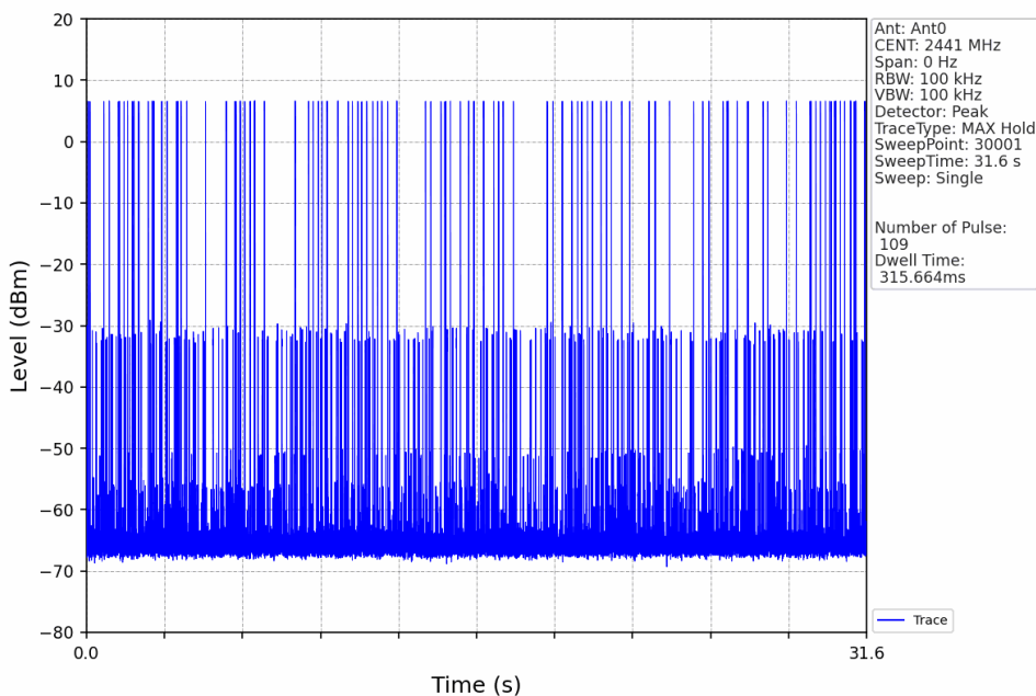
Pi/4DQPSK_2DH5_HOPP_Ant0_NTNV
