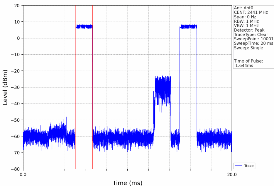
Pi/4DQPSK_2DH3_HOPP_Ant0_NTNV
