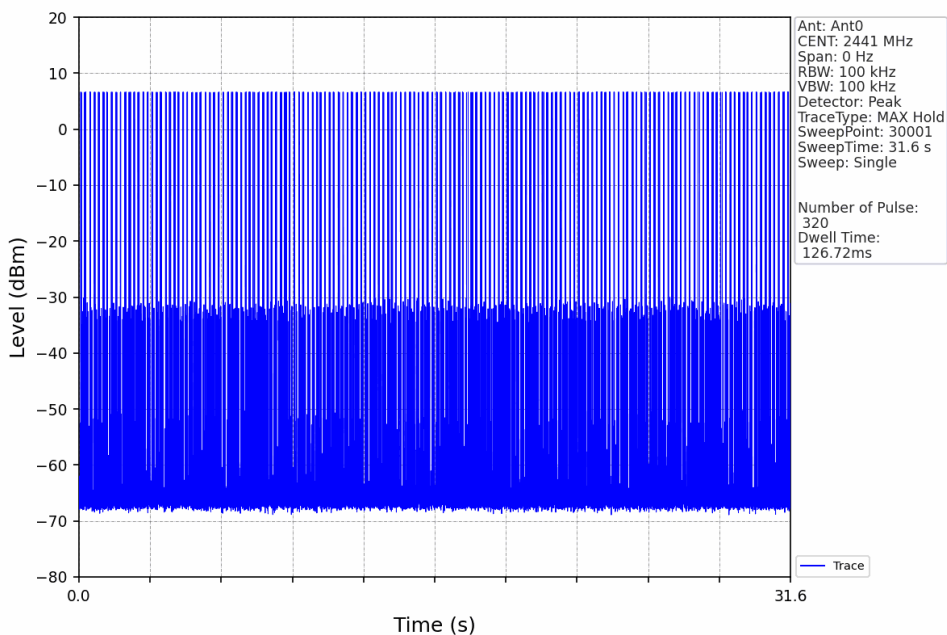
Pi/4DQPSK_2DH1_HOPP_Ant0_NTNV
