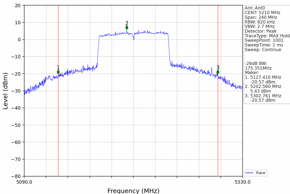
802.11ax(HEW80)_MCH_5210MHz_RU996_Left_Ant0_NTNV
