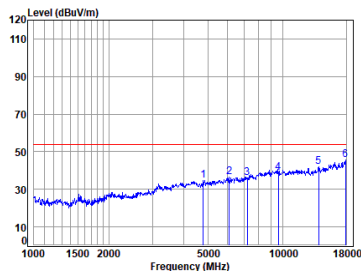
BLE_2M_TX_CH_00_Vertical-Avg
