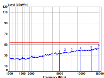
BLE_1M_TX_CH_39_Horizontal-Avg
