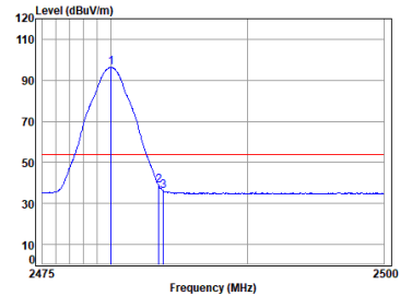
BLE_2M_TX_CH_39_Horizontal-Avg
