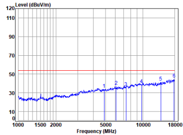
BLE_2M_TX_CH_19_Horizontal-Avg
