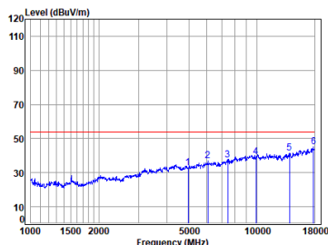
BLE_2M_TX_CH_39_Horizontal-Avg
