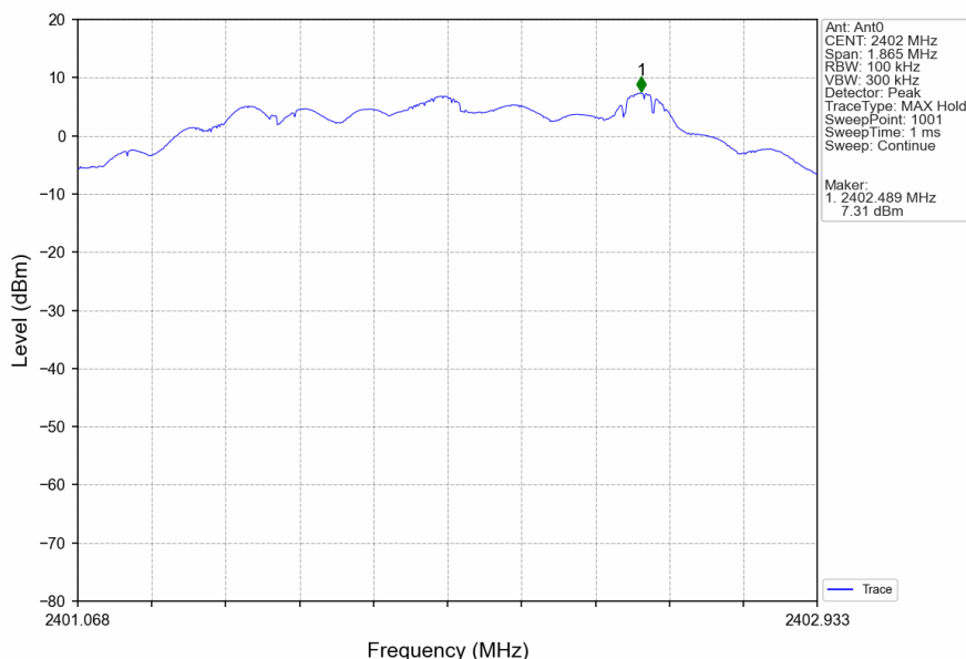
2M_LCH_2402MHz_Ant0_NTNV
