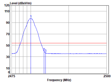
BLE_2M_TX_CH_39_Vertical-Avg
