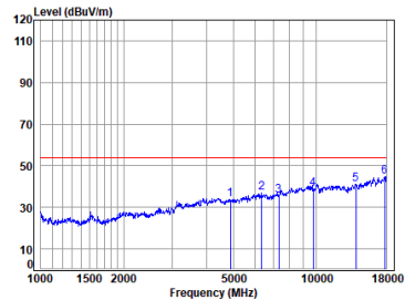
BLE_2M_TX_CH_19_Vertical-Avg
