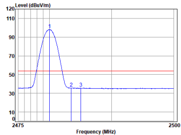
BLE_1M_TX_CH_39_Vertical-Avg
