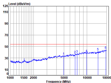
BLE_2M_TX_CH_39_Vertical-Avg
