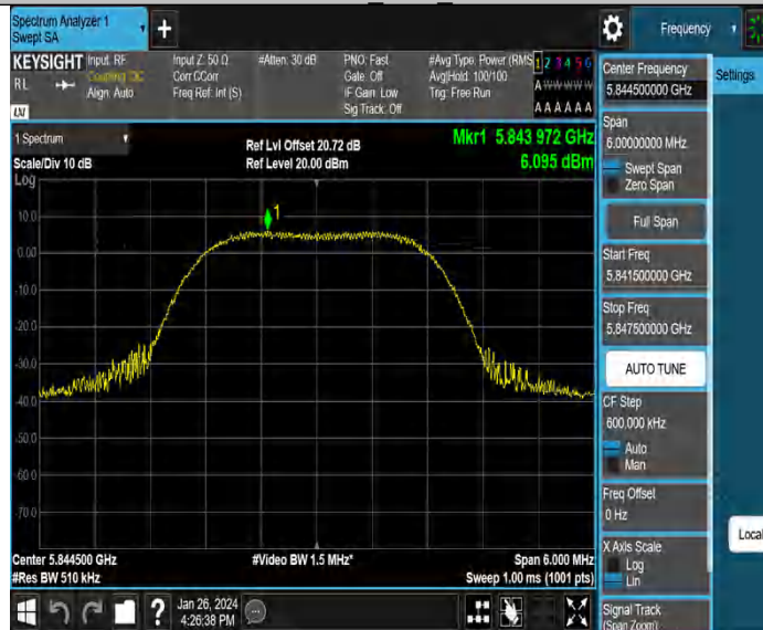
3M MIMO_Ant3_5844.5
