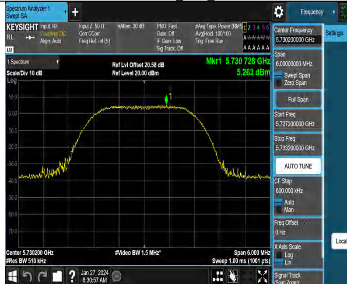
3MCA MIMO_Ant3_5730.2
