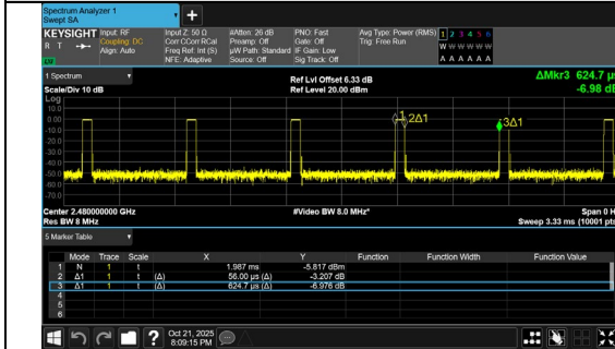
BLE 2M_Channel 39
