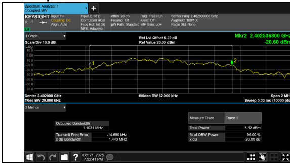
BLE 1M_Channel 0
