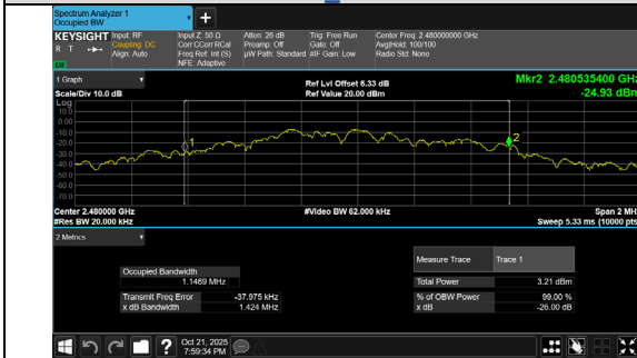
BLE 1M_Channel 39
