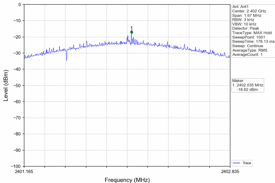
2M_LCH_2402MHz_DataRate=_Ant1_NTNV
