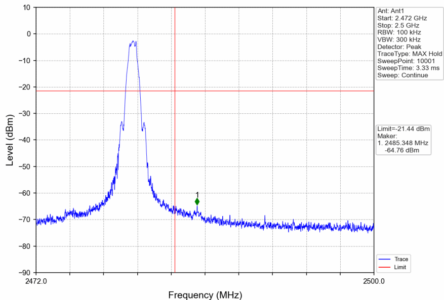
1M_HCH_2480MHz_DataRate=_Ant1_NTNV
