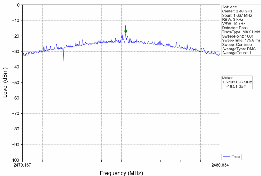
2M_HCH_2480MHz_DataRate=_Ant1_NTNV
