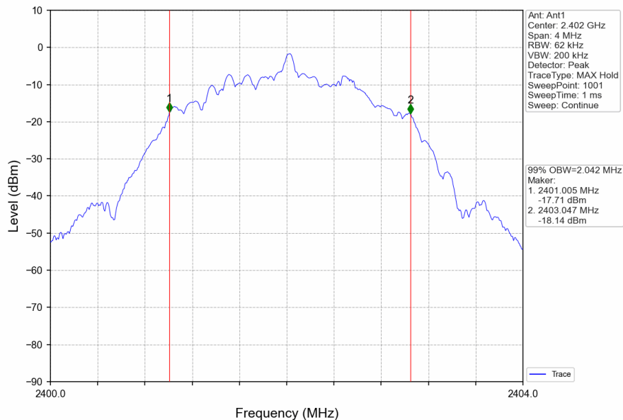
2M_LCH_2402MHz_DataRate=_Ant1_NTNV
