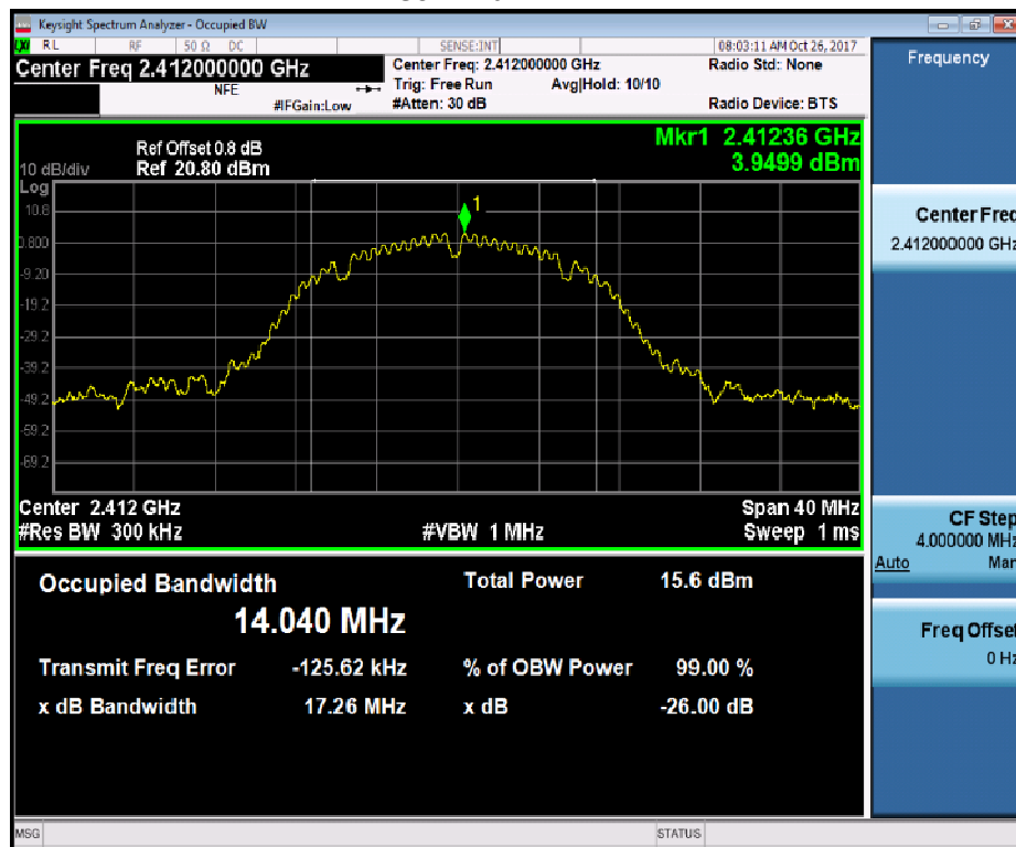
802.11b-2412MHz
