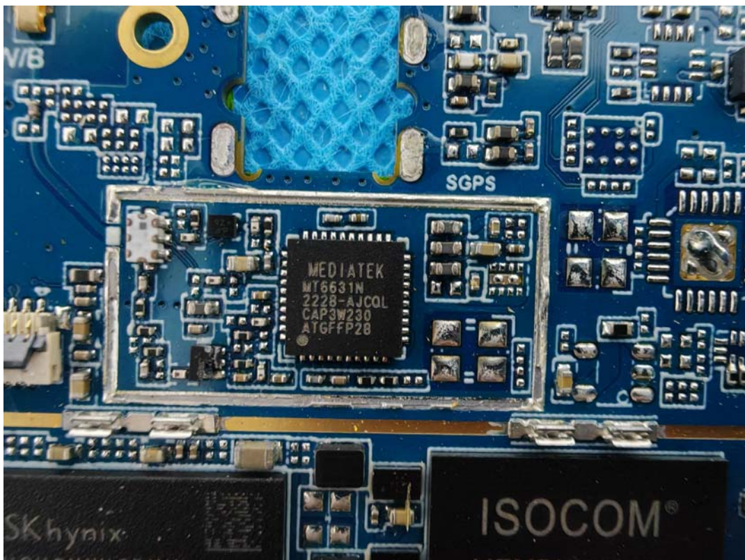
WLAN/BT/GNSS Chip
