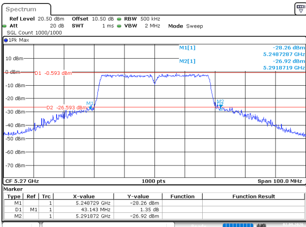
802.11ac40_5270MHz
