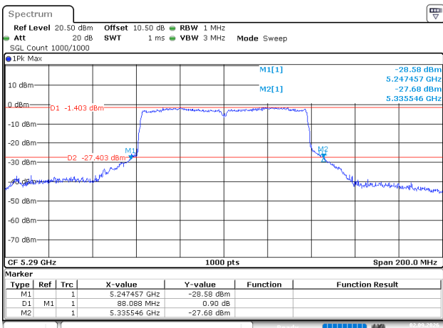
802.11ac80_5290MHz
