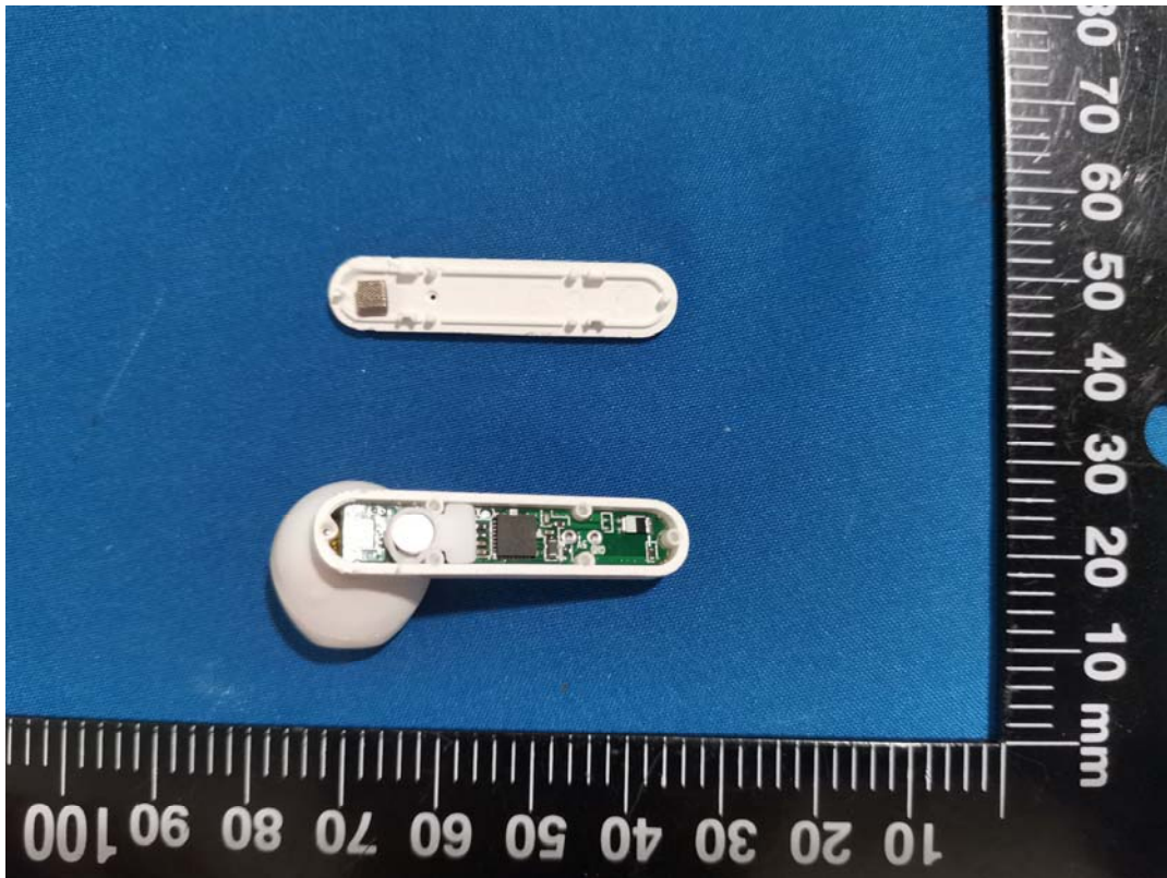
Left Unit
