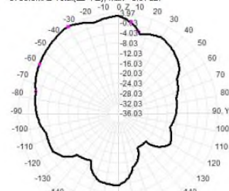
5750.0MHz Total(E2-YZ), Max= 3.97dBi
