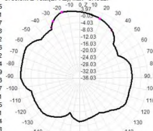
5750.0MHz Total(E1-XZ), Max= 3.49dBi
