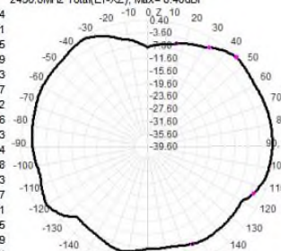
2450.0MHz Total(E1-XZ), Max= 0.40dBi
