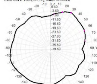
2450.0MHz Total(E2-YZ), Max= -0.05dBi
