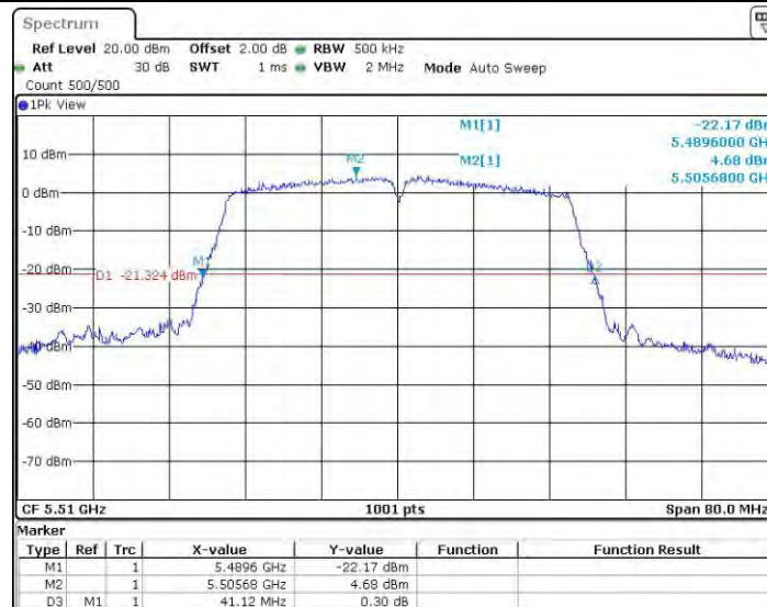
11AC40MIMO_Ant1_5510
