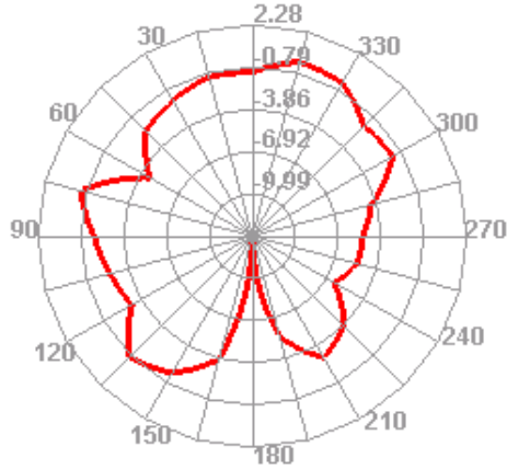
2450.000MHz E1
