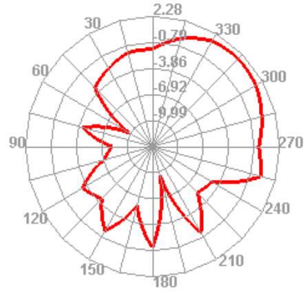
2450.000MHz E2
