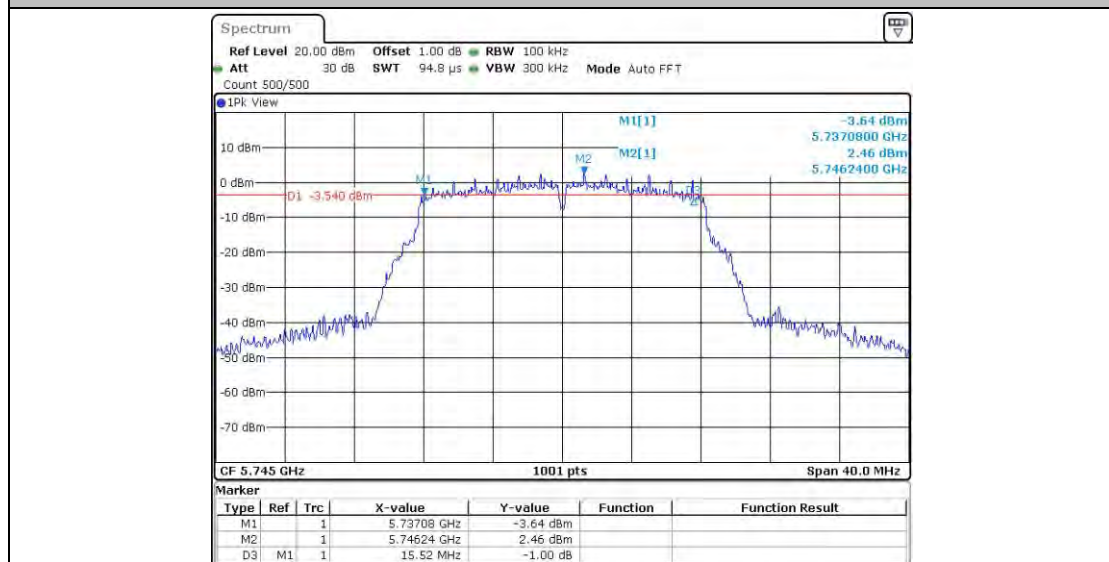
11A_Ant1_5745
