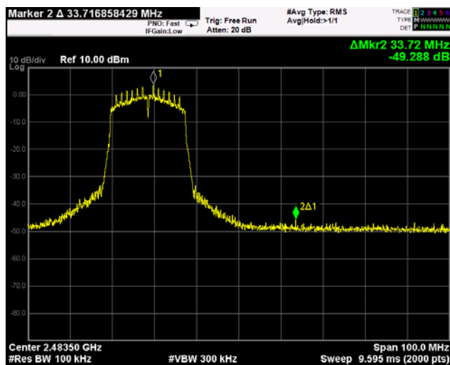
802.11n(HT40)_CH High
