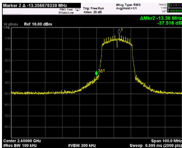
802.11n(HT40)_CH Low
