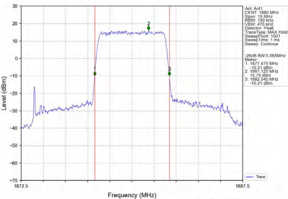
Band2_5MHz_QPSK_MCH_1880MHz_RB_25_0_NTNV
