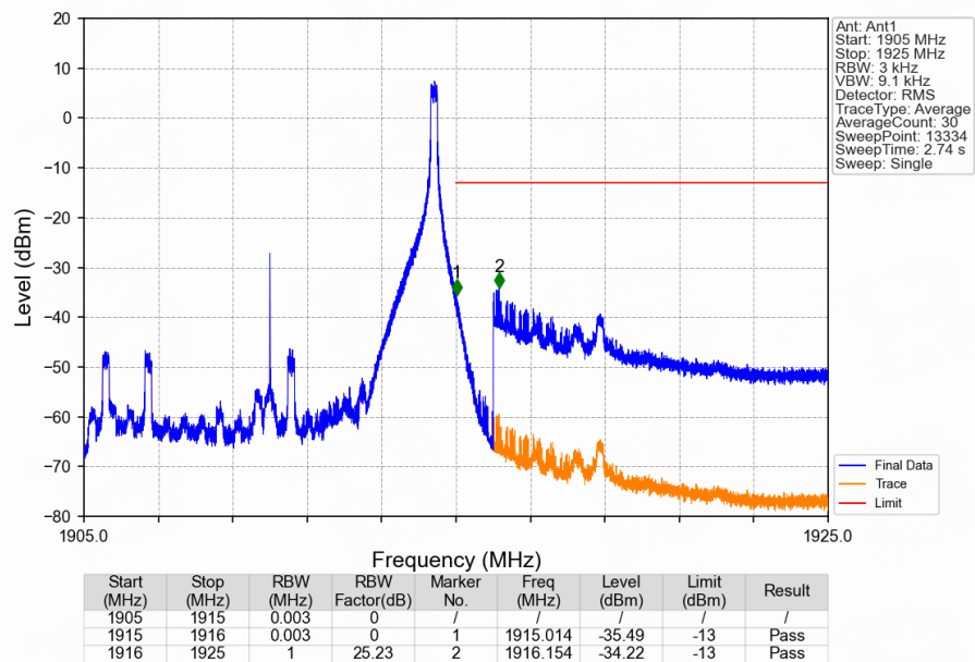
Band25 10MHz 16QAM HCH 1910MHz RB 1 49 NTNV
