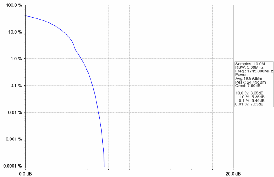
Band66_20MHz_QPSK_MCH_1745MHz_RB_100_0_NTNV
