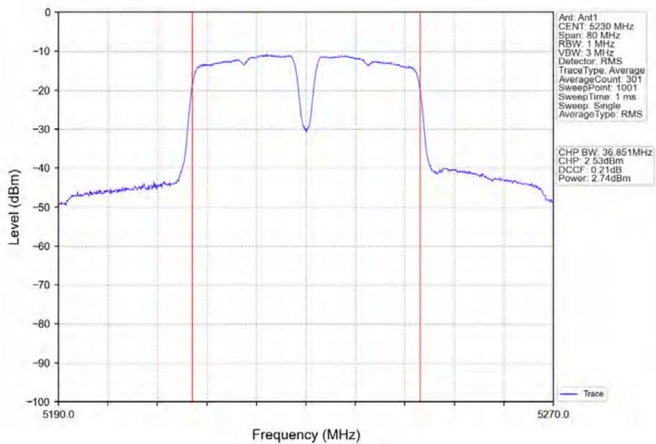
802.11ax(HEW40)_HCH_5230MHz_RU484_Left_Ant1_NTNV
