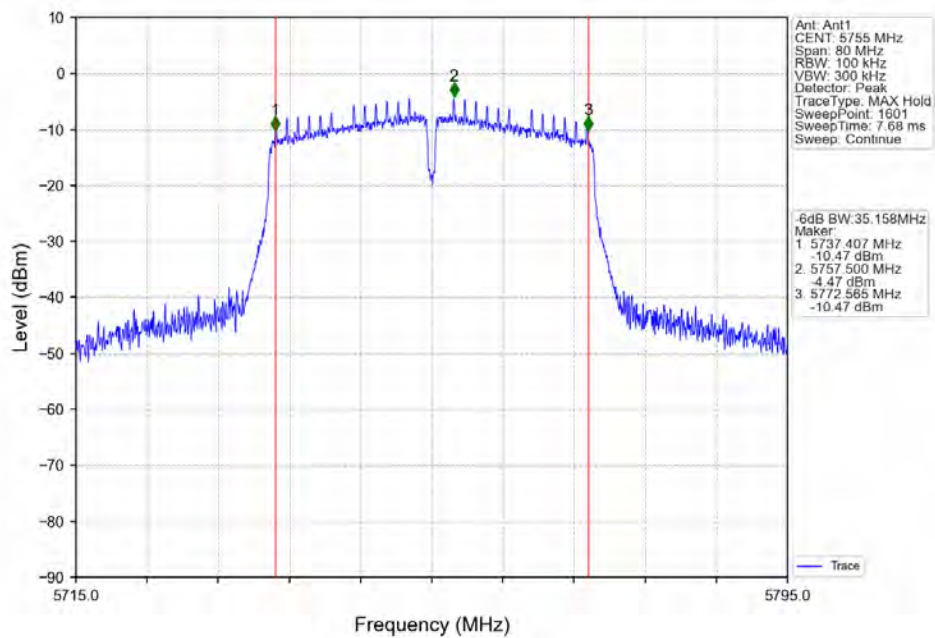
802.11ax(HEW40)_LCH_5755MHz_RU484_Left_Ant1_NTNV
