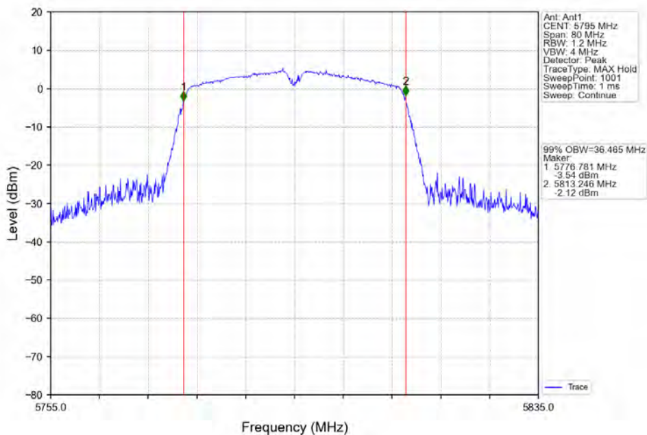
802.11ax(HEW40)_HCH_5795MHz_RU484_Left_Ant1_NTNV
