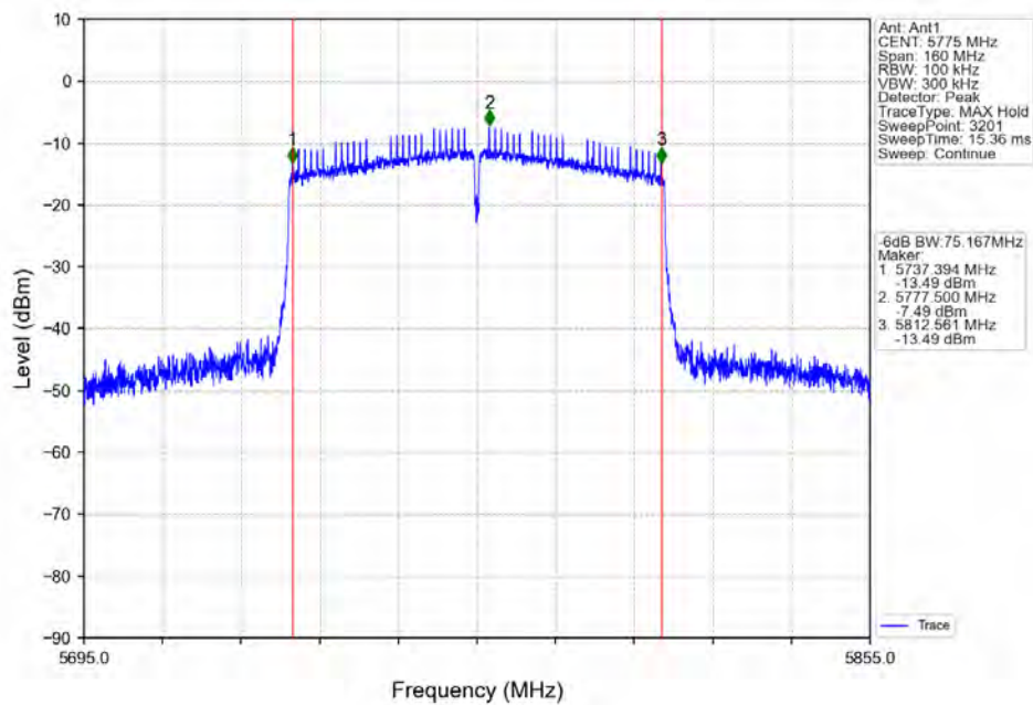
802.11ax(HEW80)_MCH_5775MHz_RU996_Left_Ant1_NTNV
