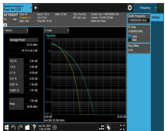
Band25-20MHz-16QAM-26365-100RB#0
