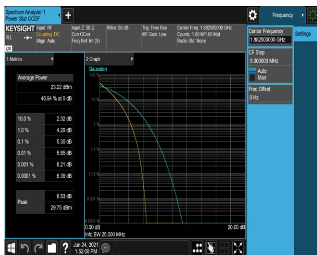
Band25-20MHz-QPSK-26365-100RB#0
