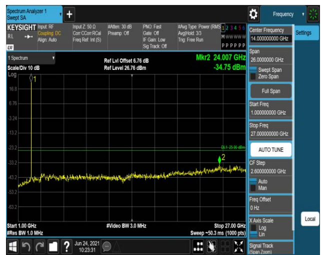
Band7-20MHz-QPSK-21100:1000~27000MHz
