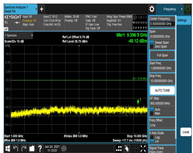
Band12-10MHz-QPSK-23095:1000~10000MHz
