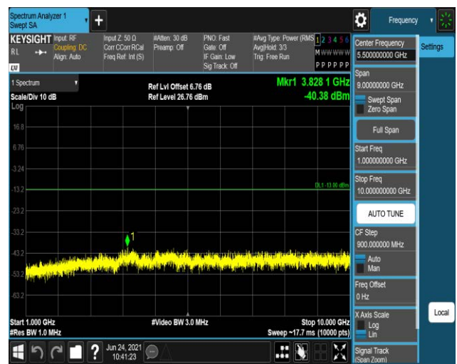
Band12-1.4MHz-QPSK-23095:1000~10000MHz
