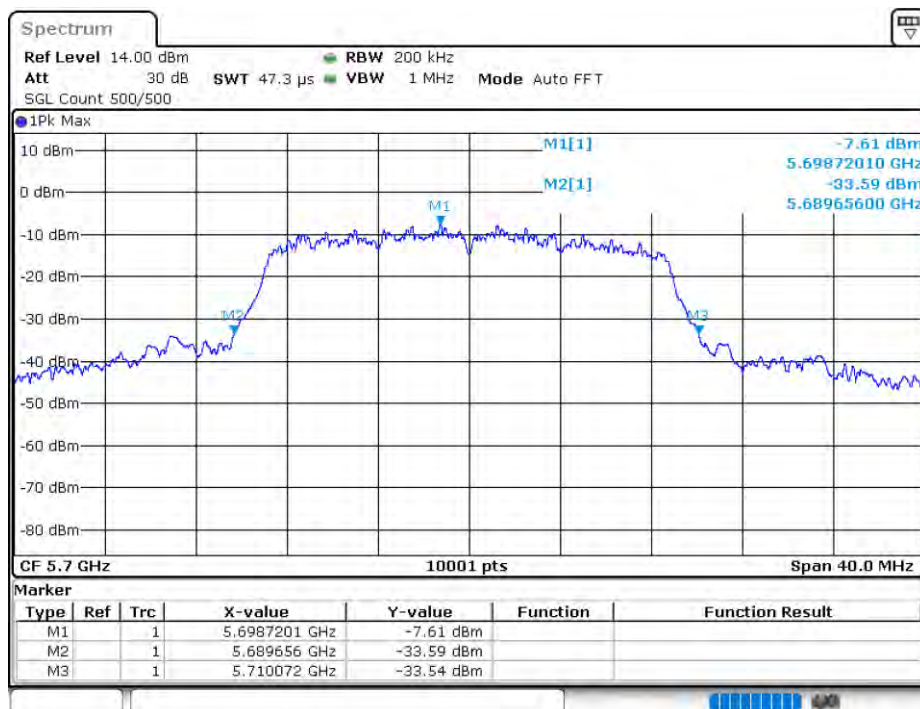
-26 dB BW NVNT 802.11n(HT20) 5700MHz Ant1
