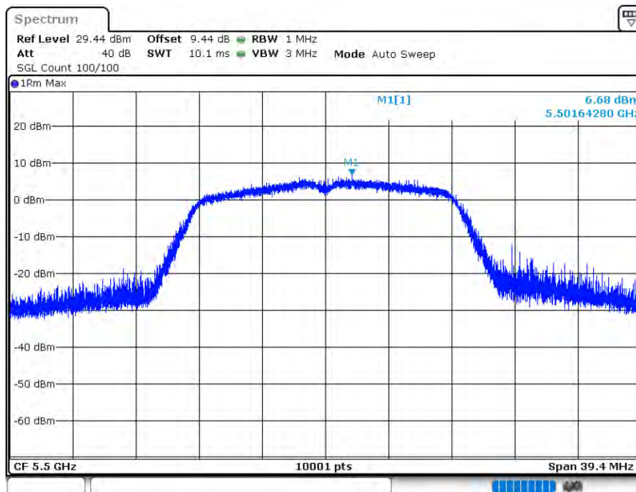
PSD NVNT 802.11a 5500MHz Ant1
