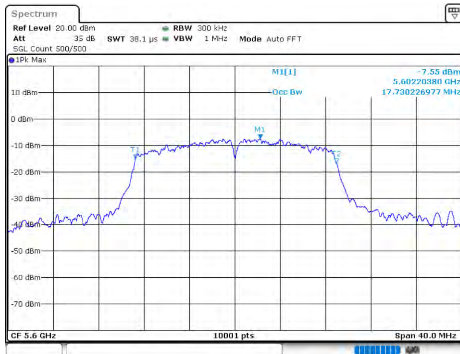
OBW NVNT 802.11ac20 5600MHz Ant1
