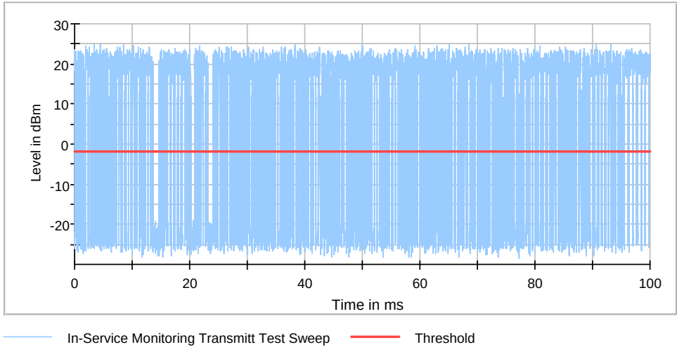
802.11a 5260 MHz_Ant 0+1
