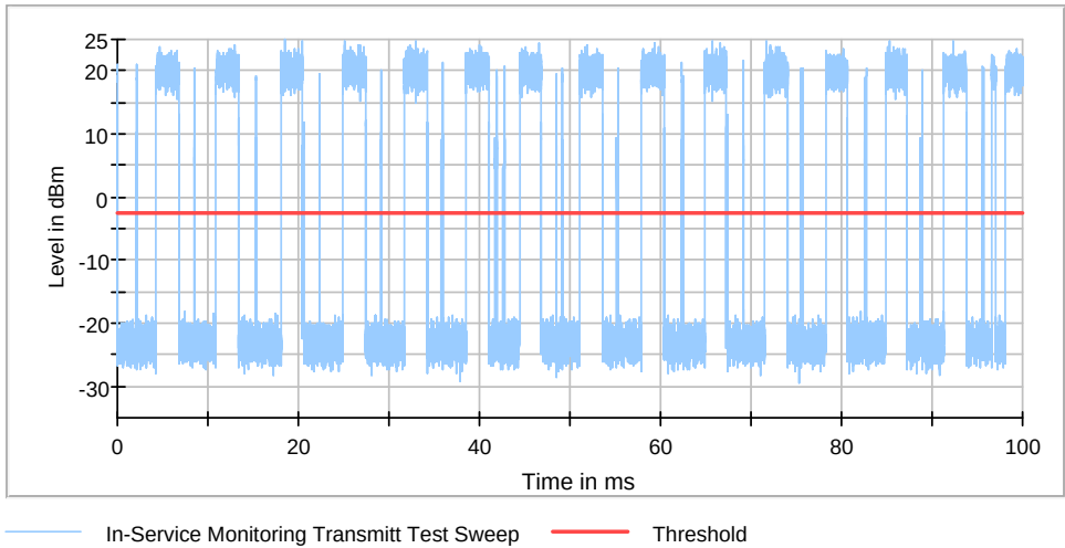
802.11n HT20 5260MHz_Ant 0+1
