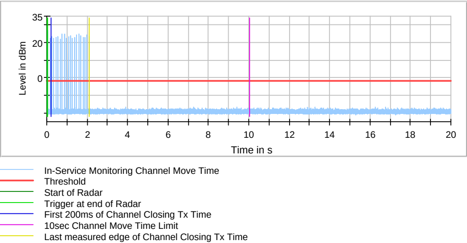
802.11a 5260 MHz_Ant 0+1
