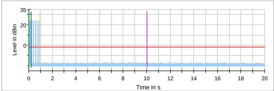
802.11n HT20 5260MHz_Ant 2
