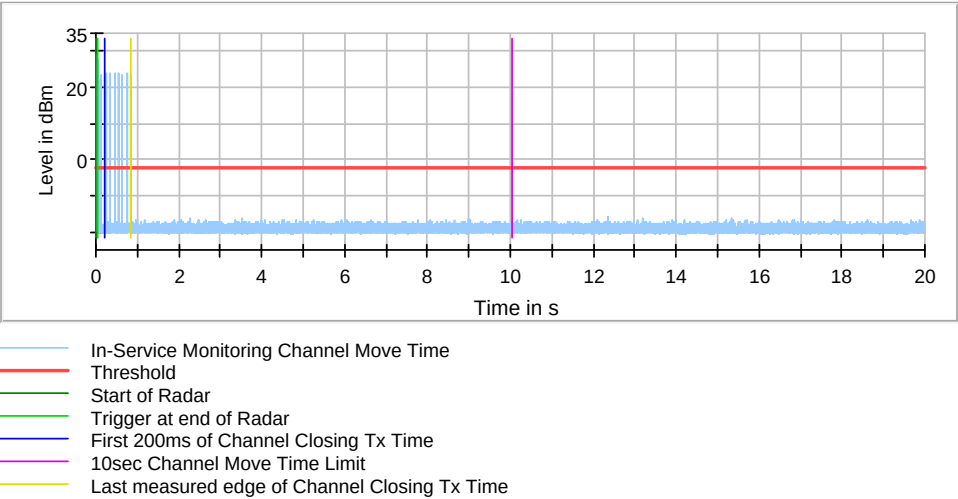
802.11ac VHT20 5260MHz_Ant 2
