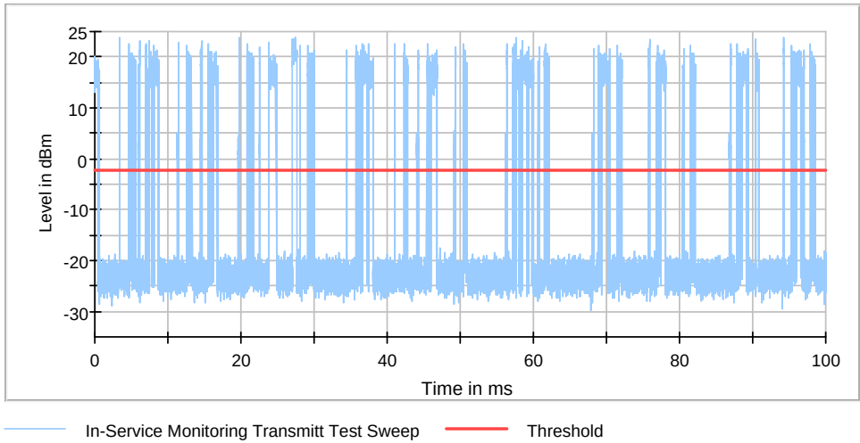
802.11ac VHT20 5260MHz_Ant 2
