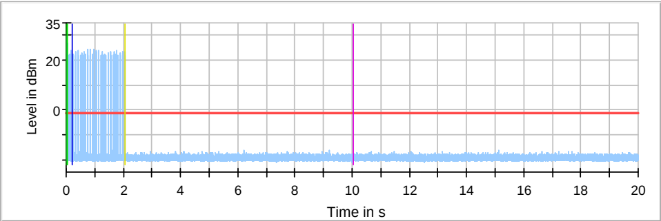
802.11ac VHT20 5260MHz_Ant 0+1
