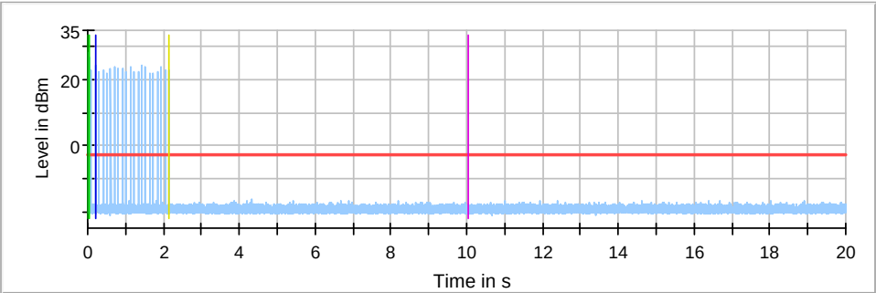
802.11n HT20 5260MHz_Ant 0+1
