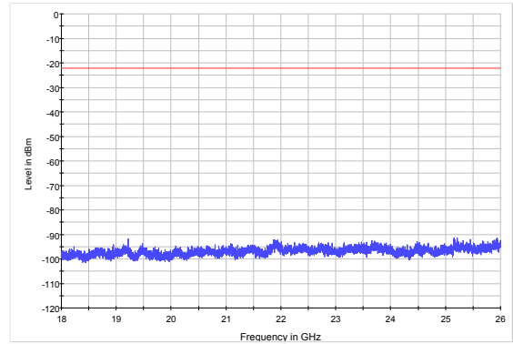
BLE CH0 18GHz to 26GHz
