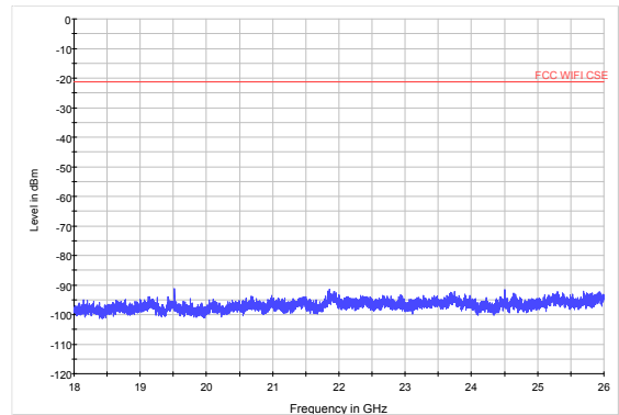
BLE CH19 18GHz to 26GHz
