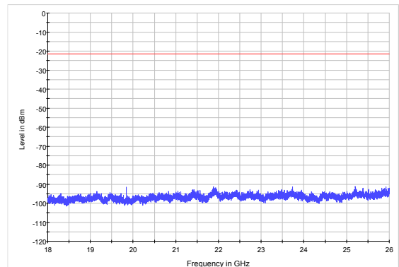
BLE CH39 18GHz to 26GHz
