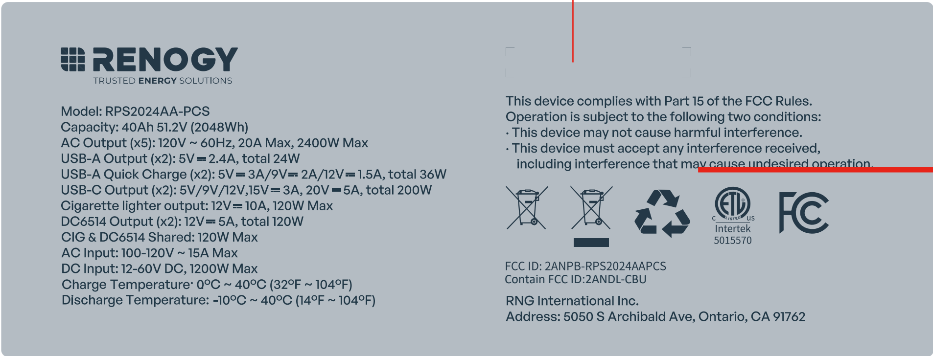
6612-02-002123 256*96mm parameter label
