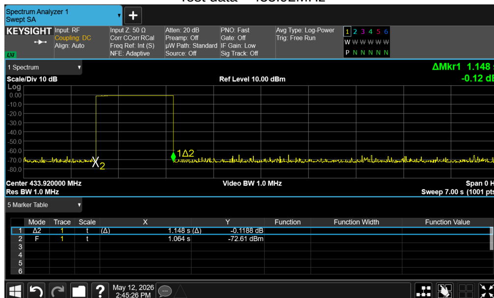
Test data—433.92MHz
