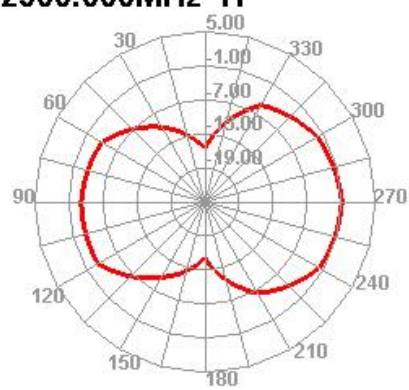
2500.000MHz E2
