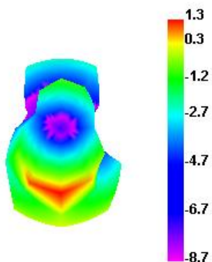
2450.000MHz E1
