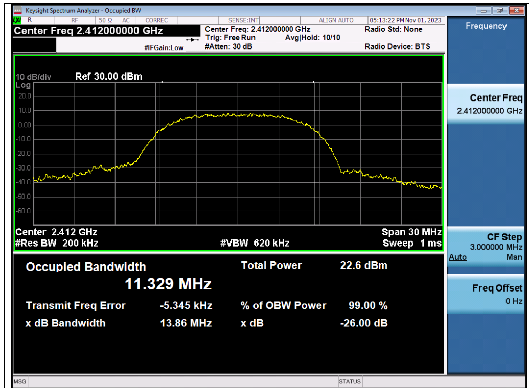
Test_Graph_802.11b_ANT1_2412_11Mbps_OBW
