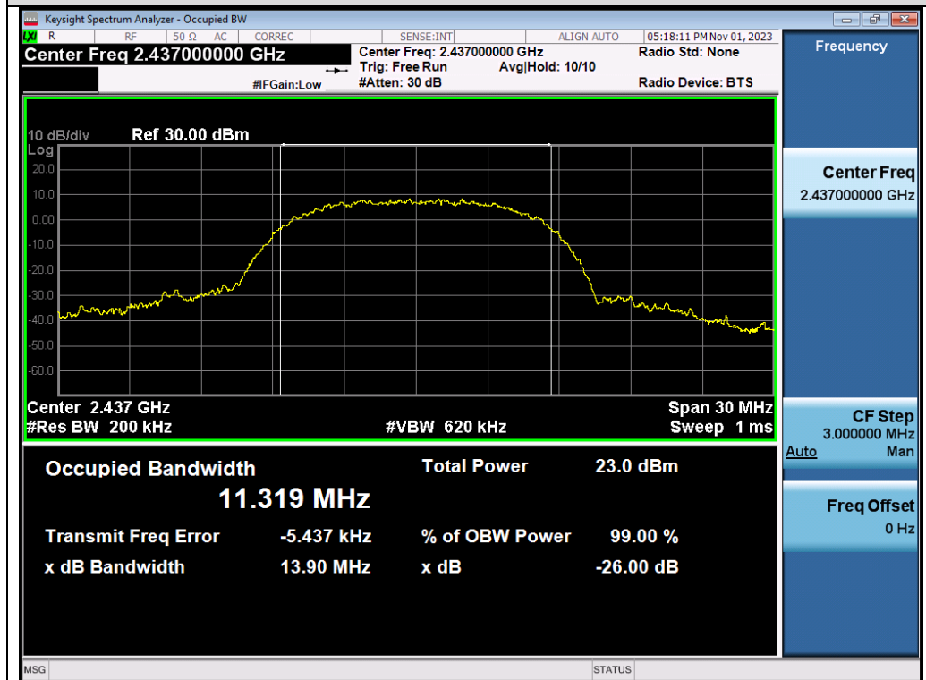
Test_Graph_802.11b_ANT1_2437_11Mbps_OBW
