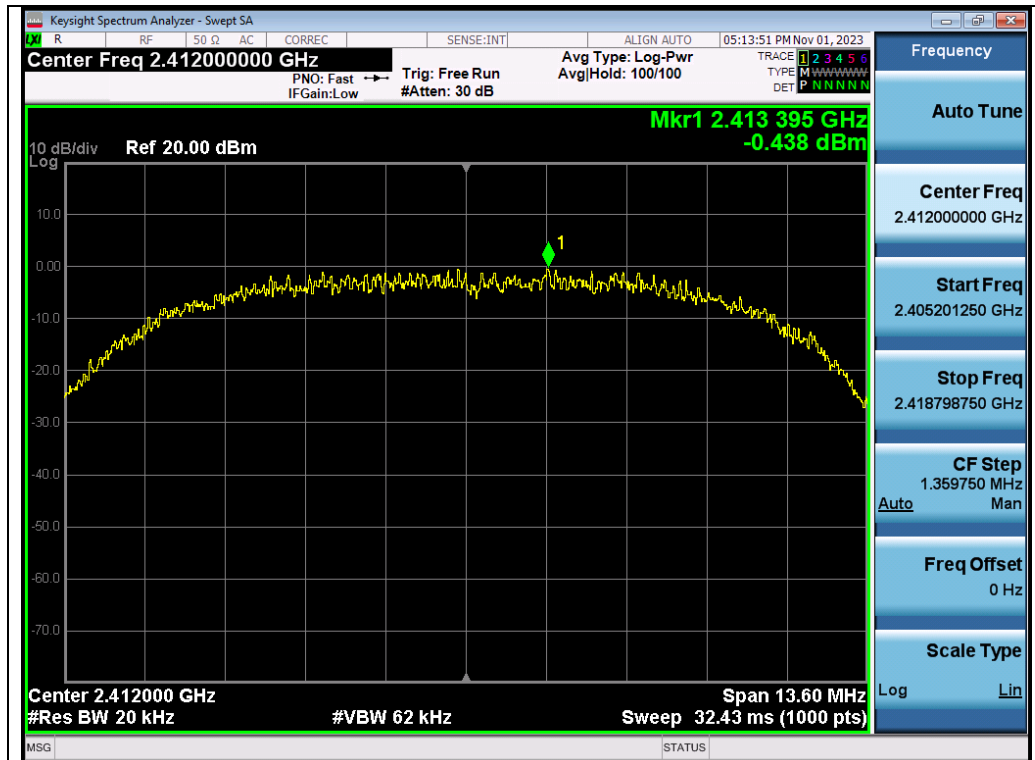
Test_Graph_802.11b_ANT1_2412_11Mbps_PSD
