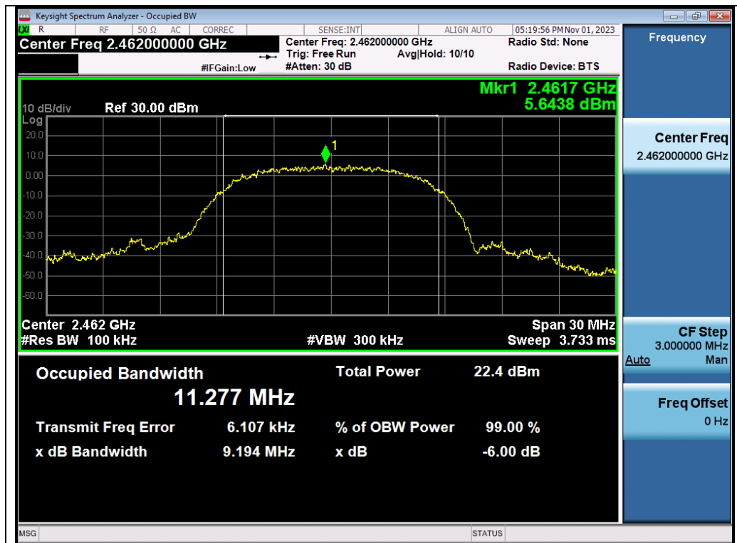
Test_Graph_802.11b_ANT1_2462_11Mbps_DTSBW
