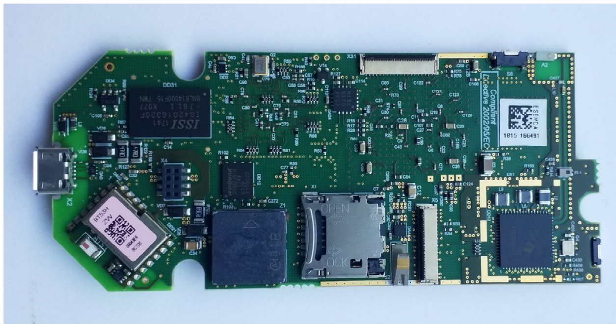
Main PCA Bottom view
