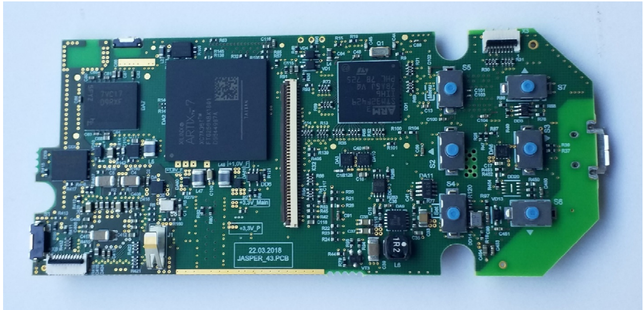
Main PCA Top view
