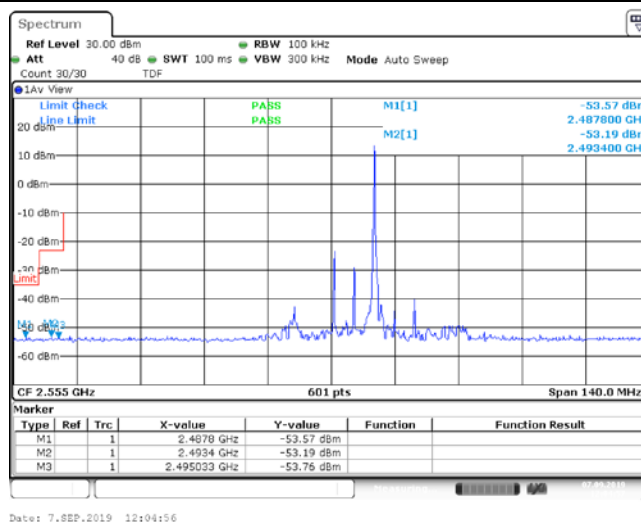
Band41_10MHz_QPSK_40290_50RB#0
