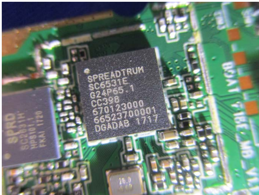
EUT –GSM&BT Chip View
