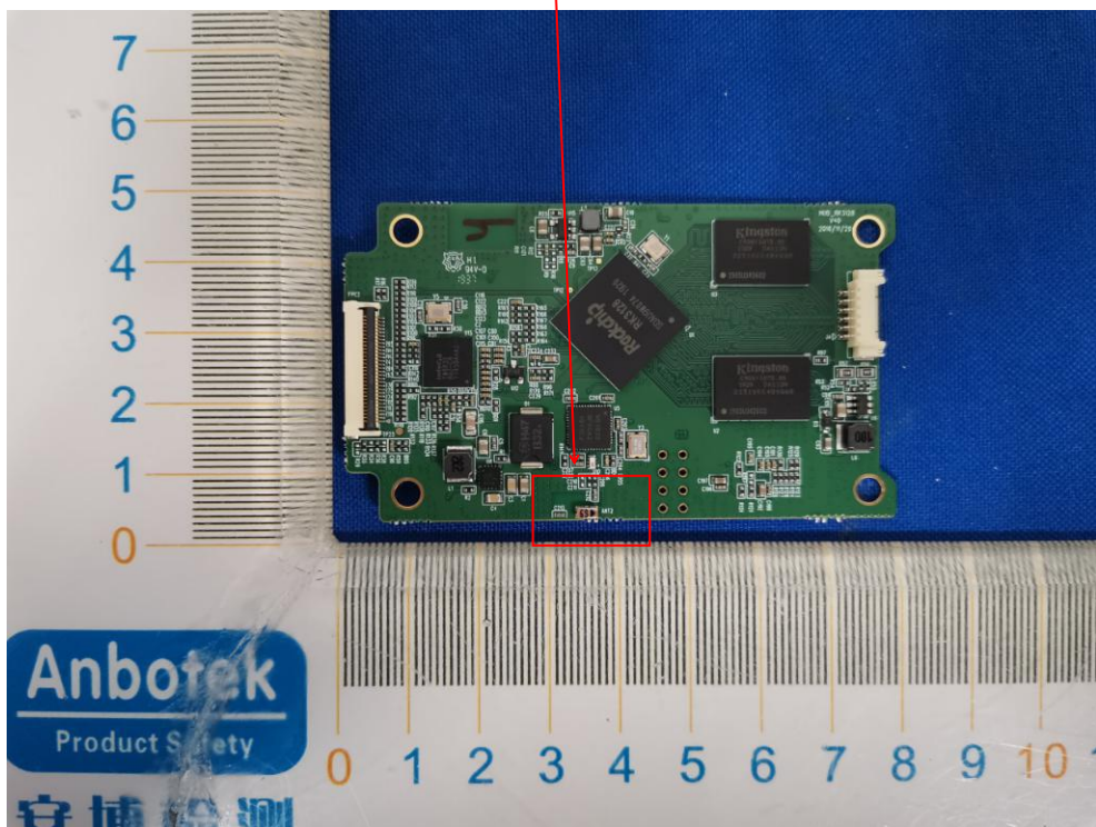
BT 1 ANT
