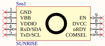
CO2 Pin Headers
