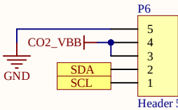
CO2 Pin Headers
